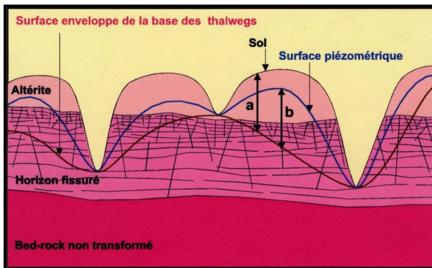
Figure 113 : Détermination des paramètres a et b nécessaire à l'estimation de la surface piézométrique (Wyns, 1999)
