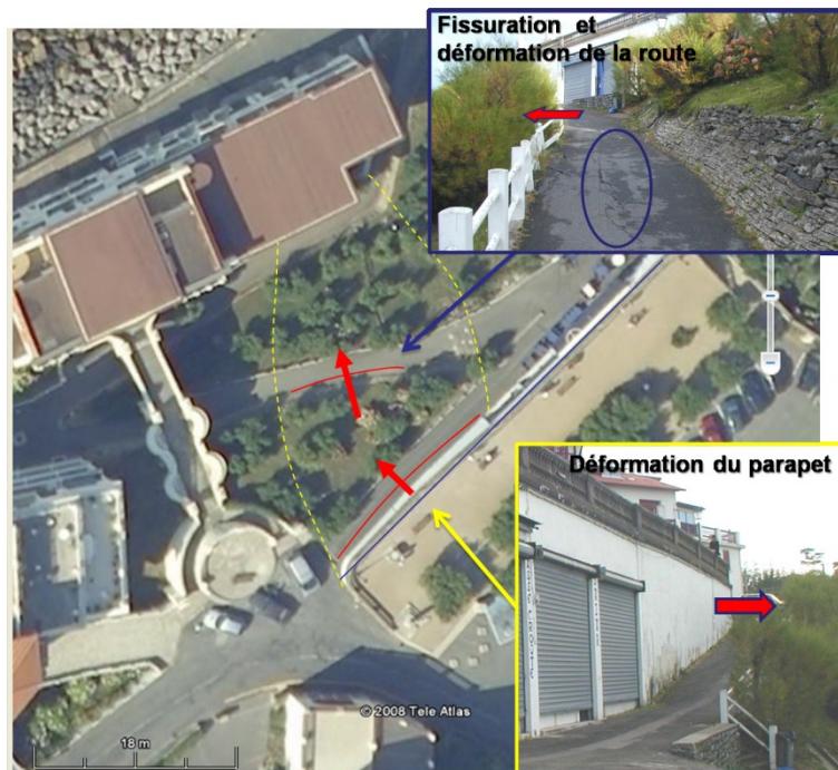
Figure 132 : Indices de fluage en centre ville de Guéthary (Image satellite Google Earth 2008)
