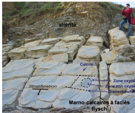
Figure 39 : L'horizon karstifié : familles de discontinuités dont les épontes sont oxydées
