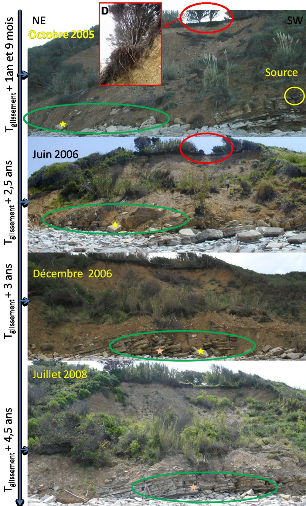
Figure 128 : Evolution du glissement (2/2)
