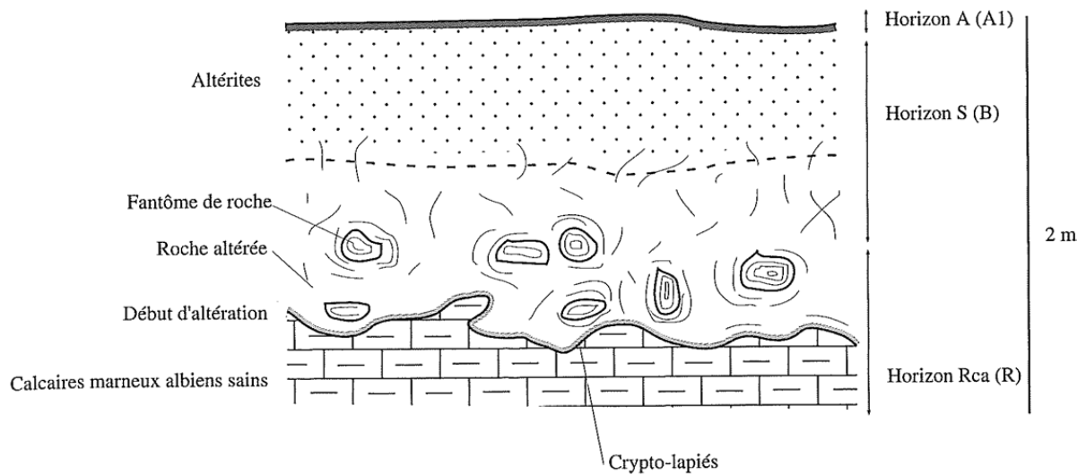
Figure 26 : Profil d'altération des calcaires marneux albiens dans le massif des Arbailles (Vanara, 2000). Dénomination des différents horizons selon la nomenclature du Référentiel Pédologique (AFES, 1995) et du Référentiel de la Commission de Pédologie et de Cartographie des sols (CPCS, 1967 ; entre parenthèses)
