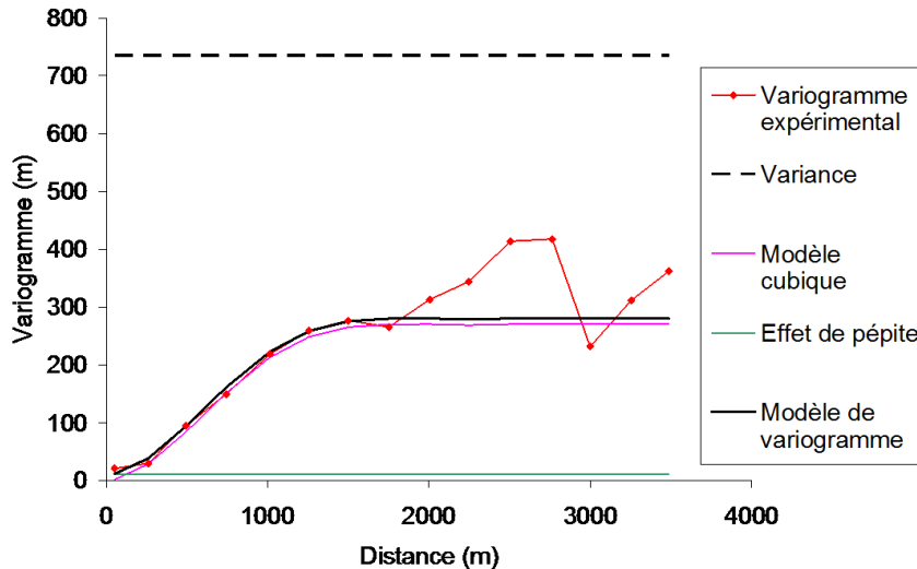
Figure 63 : Variogramme expérimental calculé à partir des données exactes de l'altitude du mur des altérites (MEXAALTE) et modèle de variogramme (nombre de paires minimum utilisé pour le calcul : 197)
