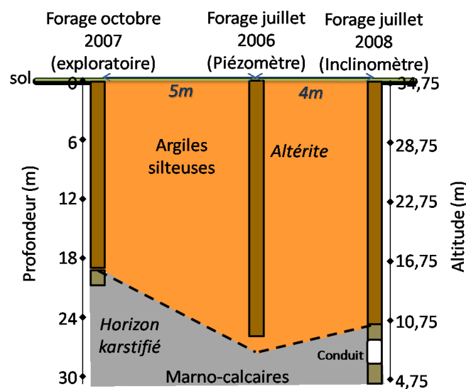
Figure 109 : Coupe schématique de la Muserie
