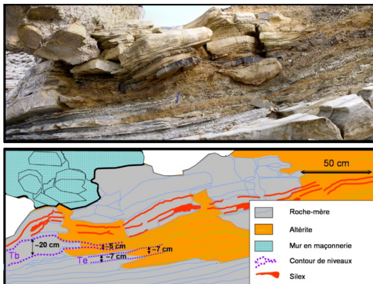
Figure 31 : Passage de la roche-mère à l'altérite parallèle à la stratification : photographie (en haut) et interprétation (en bas). On remarque, en plus de la conservation de la stratification, une perte de volume des termes basaux des turbidites
