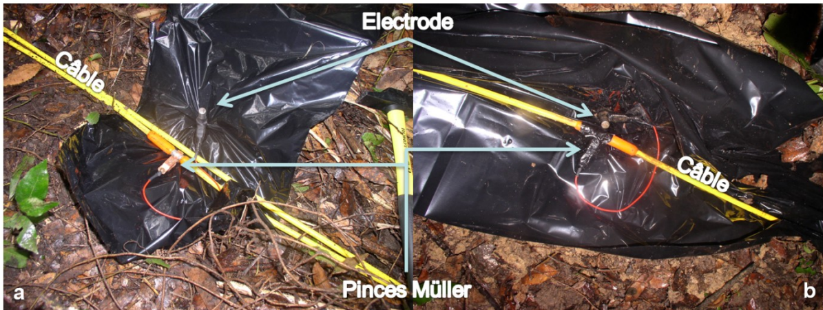
Figure 1 : Dispositif de tomographie électrique : connexion des électrodes au câble : a. avant protection des connectiques b. protection avec un adhésif thermocollant imperméable
