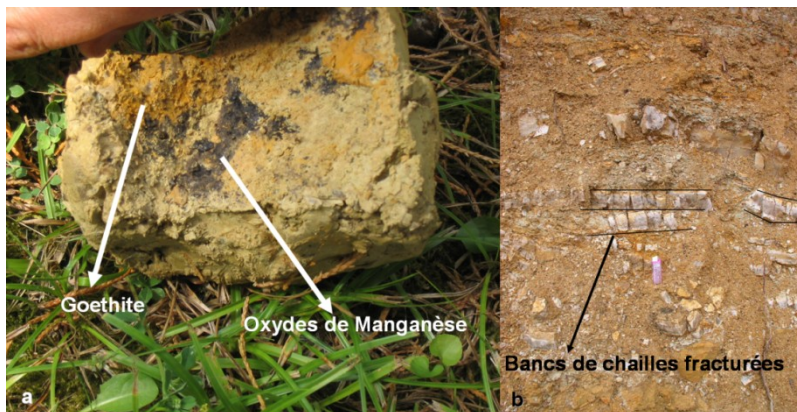
Figure 30 : a. Échantillon d'altérite du Flysch à silex de Guéthary : les oxydes de fer (goéthite) colorent la roche dans des teintes ocres et les oxydes de manganèse en noir ; b. Bancs de chailles blanchies et fracturées
