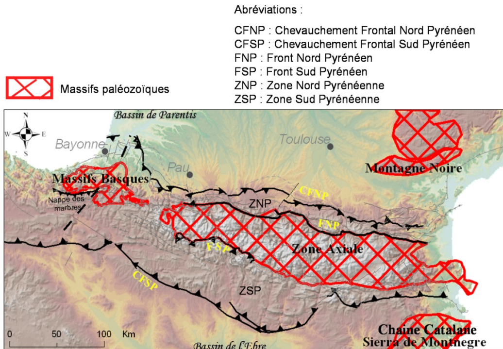
Figure 4 : Structures majeures du système pyrénéen (carte réalisée d'après les cartes structurales de Razin, 1989, Bîteau et Canérot, 2007, et Choukroune et Séguret, 1973)
