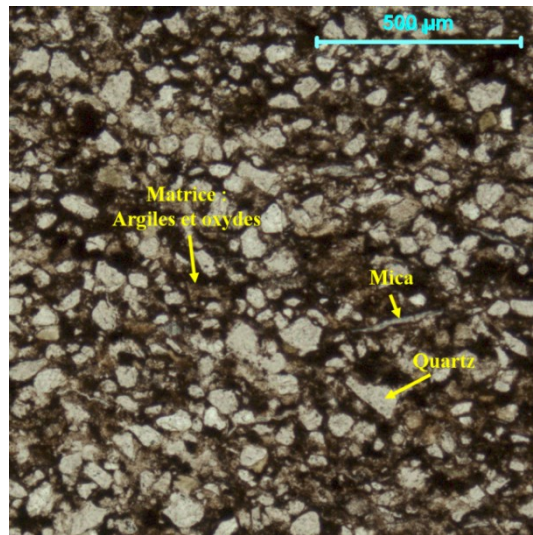
Figure 48 : Section perpendiculaire à la stratification d'un niveau gréseux d'altérite (grauwacke quartzeuse ; échantillon A29, Annexe 4) vue au microscope optique en lumière polarisée non analysée (LPNA ; \times 50 ; grossissement de l'objectif : \times 10 et grandissement de l'oculaire : \times 5 )
