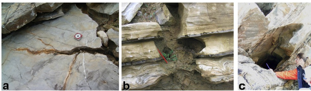
Figure 40 : a. Evolution latérale de discontinuités aux épontes oxydées en conduit ; b : conduit de type karstique remplis d'altérite en place ; c. Conduit karstique évidé localisé dans un terme grossier des marno-calcaires à faciès flysch
