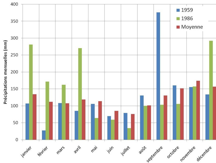
Figure 133 : Précipitations mensuelles en 1959 et en 1986 et moyennes mensuelles entre 1921 et 2008 à Socoa (Source : Météo France, 2008)
