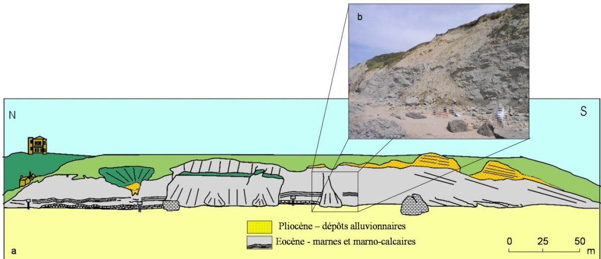
Figure 22 : a. Panorama des falaises éocènes d'Ilbarritz (Bidart) ; b. Coulée boueuse survenue en 2004
