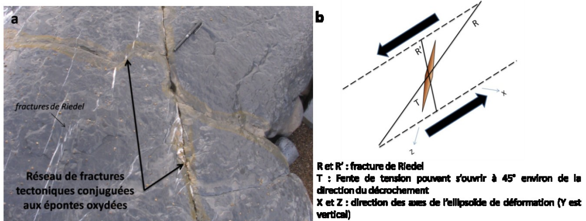
Figure 38 : a. Dalle de marno-calcaire à faciès flysch comportant des fractures tectoniques (remplissage calcitique blanc et fractures de Riedel) aux épontes non oxydées et d'autres caractérisées par des épontes oxydées ; b. Schéma de principe du modèle de Riedel en décrochement sénestre (d'après Foucault et Raoult, 2000)
