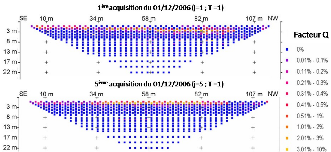
Figure 3 : Superposition des valeurs du facteur Q des acquisitions j=1 et 5 du 01/12/2006 (test T=1) et de la pseudo-section
