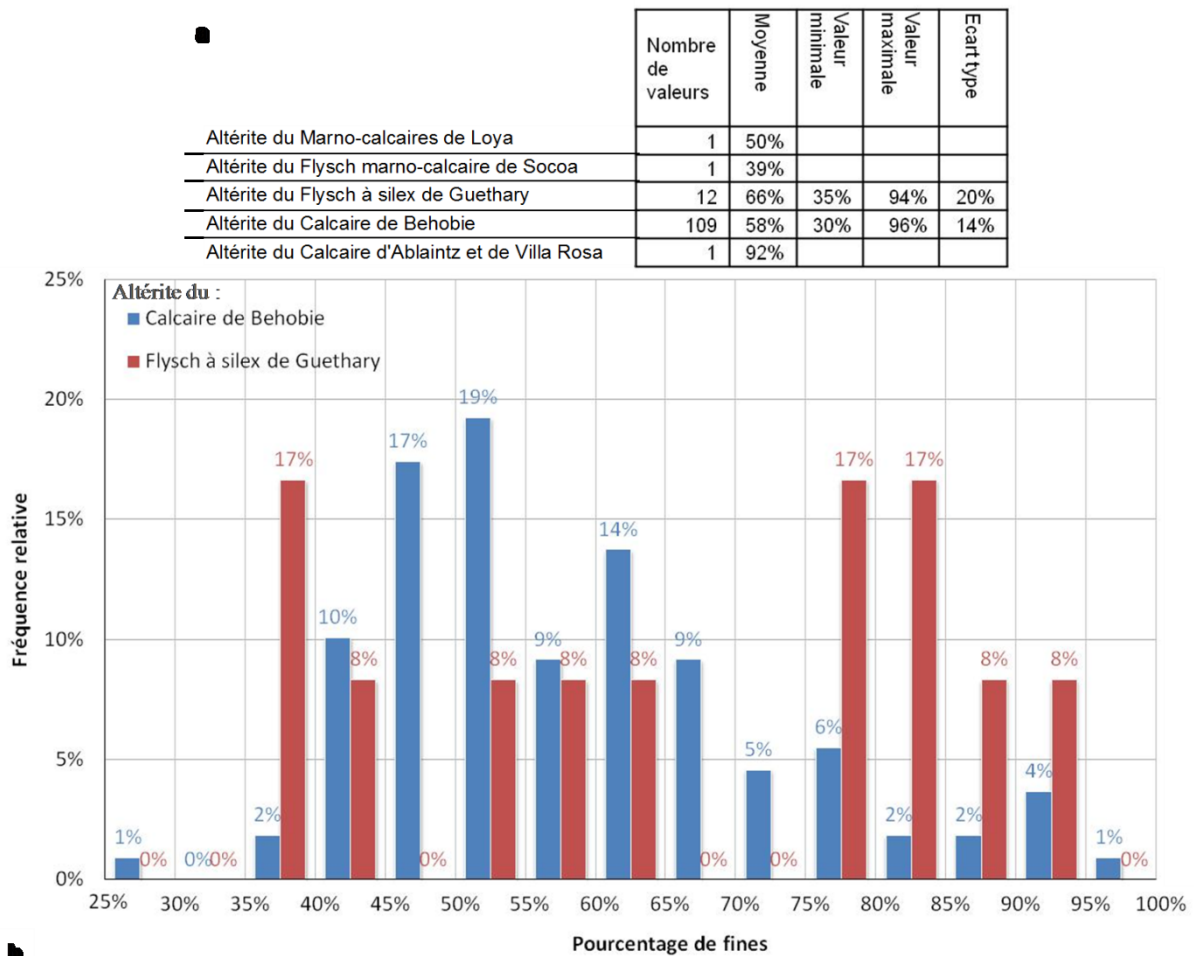
Figure 84 : a. Paramètres statistiques du pourcentage de la fraction fine (<80 μm) dans les altérites des marno-calcaires à faciès flysch du Cénomanién supérieur au Campanien supérieur ; b. Distribution du pourcentage de la fraction fine des altérites du Calcaire de Béhobie et du Flysch à silex de Guéthary
