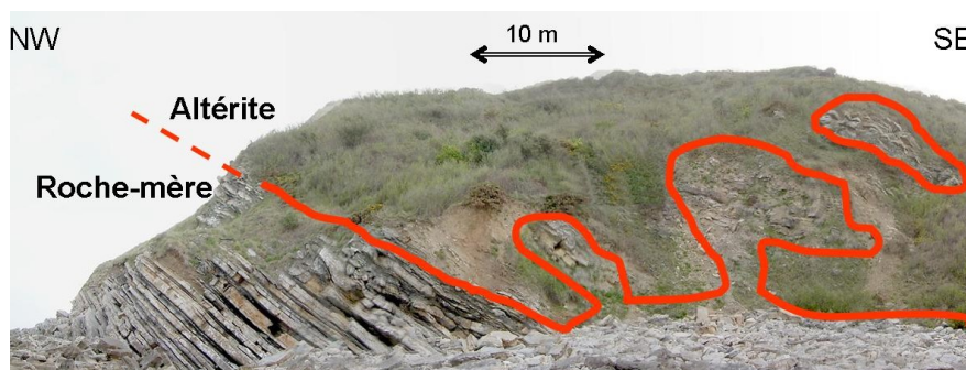
Figure 41 : Exemple de la complexité de la géométrie de l'interface de la roche-mère et de l'altérite à l'échelle des reliefs côtiers (Eromardie Nord ; Saint-Jean-de-Luz)
