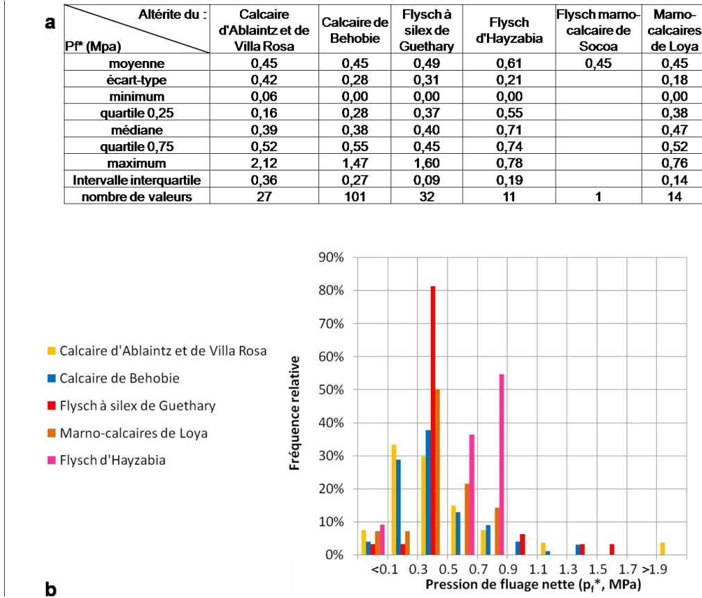
Figure 89 : Paramètres statistiques (a) et distribution (b) des pressions de fluage nettes ( p_f^* , en MPa) par altérite
