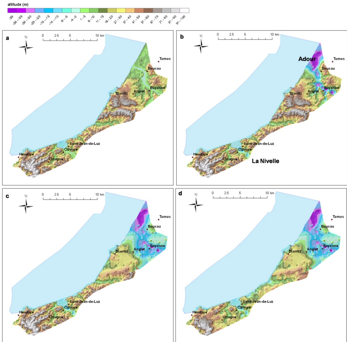
Figure 65 : a. Surface topographique ; b : Surface obtenue après suppression des alluvions récentes (FZ) ; c : Surface obtenue après suppression des alluvions récentes (FZ) et des formations plio-quadernaires (PLIO) ; d : Surface obtenue après suppression des alluvions récentes (FZ), des formations plio-quadernaires (PLIO) et des altérites (ALTE), c'est aussi le toit du substratum et le mur des altérites dans la limite de leur présence
