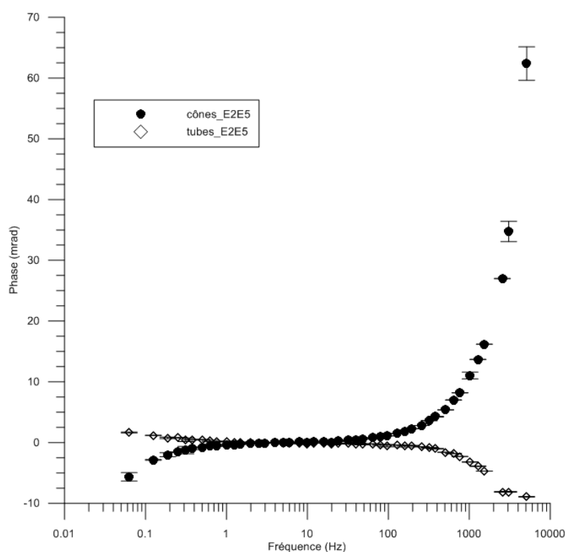
FIGURE 0-15 : PHASE DE LA RÉSISTIVITÉ COMPLEXE D'UNE COLONNE DE SABLE SATURÉ, MESURÉE PAR LE GDP 32 EN MODE 16 BITS, POUR LE COUPLE E2E5, SUR LES ÉLECTRODES DE TYPE CÔNE (RONS PLEINS) ET DE TYPE TUBE (LOSANGES VIDES). LES BARRES D'ERREUR CORRESPONDENT UN ÉCART TYPE CALCULÉ SUR 6 MESURES PAR FRÉQUENCE.
