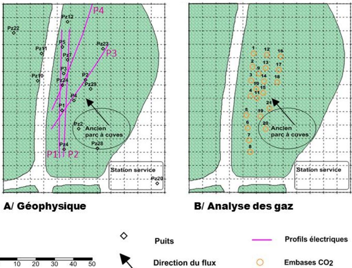
FIGURE VI-4 : CARTES DE L'EMPLACEMENT A/ DES 4 PROFILS ÉLECTRIQUES ET B/ DES 21 EMBASES UTILISÉES POUR POSER LA CHAMBRE DU SPIRIT, POUR LA CAMPAGNE DE MESURES PRÉLIMINAIRES (GÉOPHYSIQUE : MAI 2012, GAZ : SEPTEMBRE 2013).
