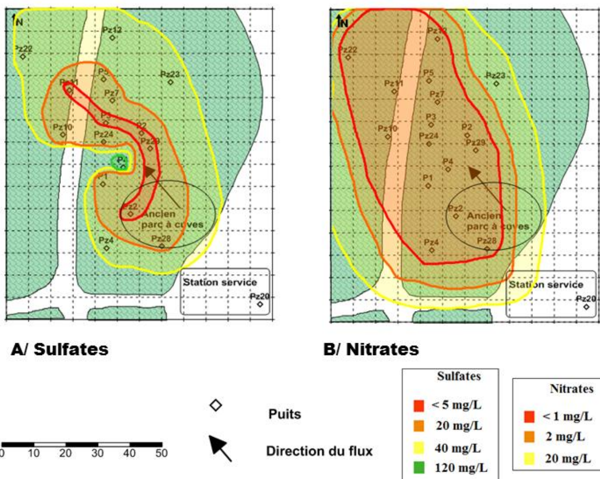
FIGURE VI-3 : CARTES DES CONCENTRATIONS EN ACCEPTEURS D'ÉLECTRONS DANS LES PUIITS DE SURVEILLANCE (SEPTEMBRE 2013) : A/ SULFATES ET B/ NITRATES. L'ANCIEN PARC À CUVES CORRESPOND À LA ZONE SOURCE DE LA POLLUTION, ET LA FLÈCHE INDIQUE LE FLUX DE DIRECTION NORD-OUEST DE LA NAPPE .
