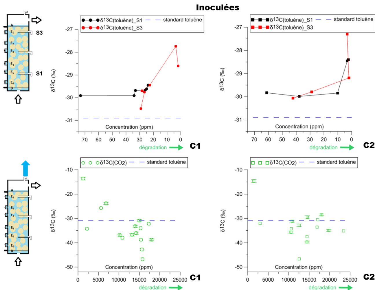
FIGURE VII-12 : EVOLUTION DE \delta^{13}\text{C}(\text{TOLUÈNE}) EN S1 ET S3 (EN HAUT) ET DE \delta^{13}\text{C}(\text{CO}_2) (EN BAS), EN FONCTION DE LA CONCENTRATION EN TOLUÈNE ET EN \text{CO}_2 , RESPECTIVEMENT, POUR LES DEUX COLONNES INOCULÉES C1 ET C2.
