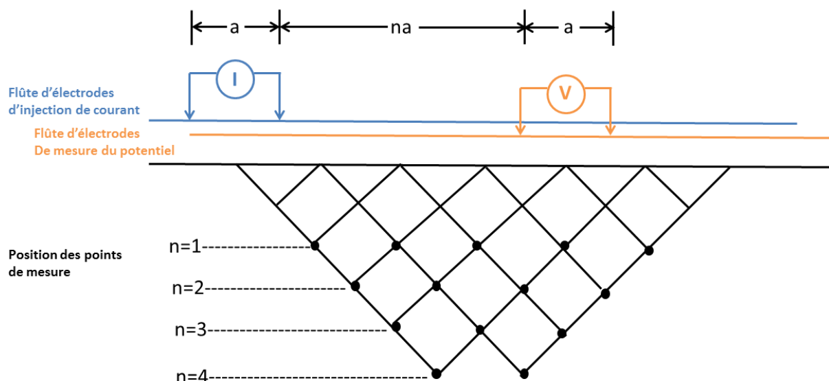
FIGURE VI-5 : CONFIGURATION DIPÔLE-DIPÔLE DU PROFIL PERMANENT : UNE FLUTE D'ÉLECTRODES EST UTILISÉE POUR L'INJECTION DE COURANT, ET UNE AUTRE FLÛTE POUR LA MESURE DU POTENTIEL.
