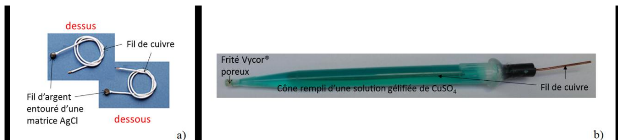
FIGURE V-7 : PHOTO DES DEUX TYPES D'ÉLECTRODES DE POTENTIEL UTILISÉES PENDANT LES EXPÉRIMENTES BIOPHY. a) ELECTRODES Ag/AgCl DU COMMERCE (WARNER INSTRUMENTS, HAMDEN, USA) ; b) ELECTRODES Cu/CuSO 4 , RÉALISÉES À PARTIR DU MODÈLE DE MAINEULT (2004).
