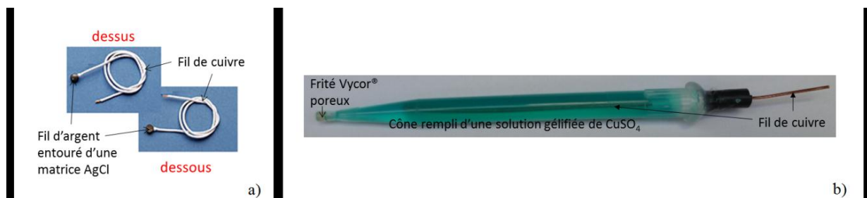
FIGURE V-7 : PHOTO DES DEUX TYPES D'ÉLECTRODES DE POTENTIEL UTILISÉES PENDANT LES EXPÉRINECES BIOPHY. a) ELECTRODES Ag/AgCl DU COMMERCE (WARNER INSTRUMENTS, HAMDEN, USA) ; b) ELECTRODES Cu/CuSO 4 , RÉALISÉES À PARTIR DU MODÈLE DE MAINEULT (2004).
