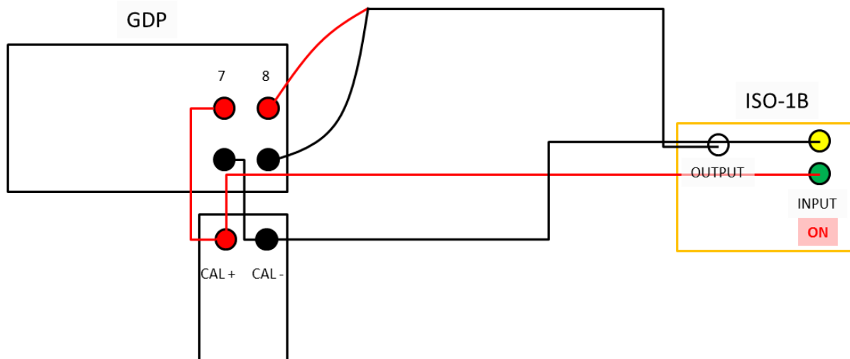
FIGURE 0-6 : SCHÉMA DU DISPOSITIF DE CALIBRATION DU GDP-32.
