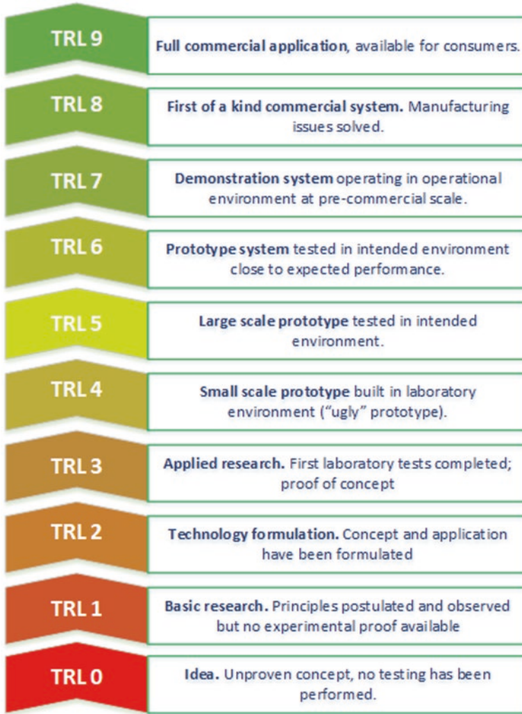
Fig. 1.4 TRL levels
