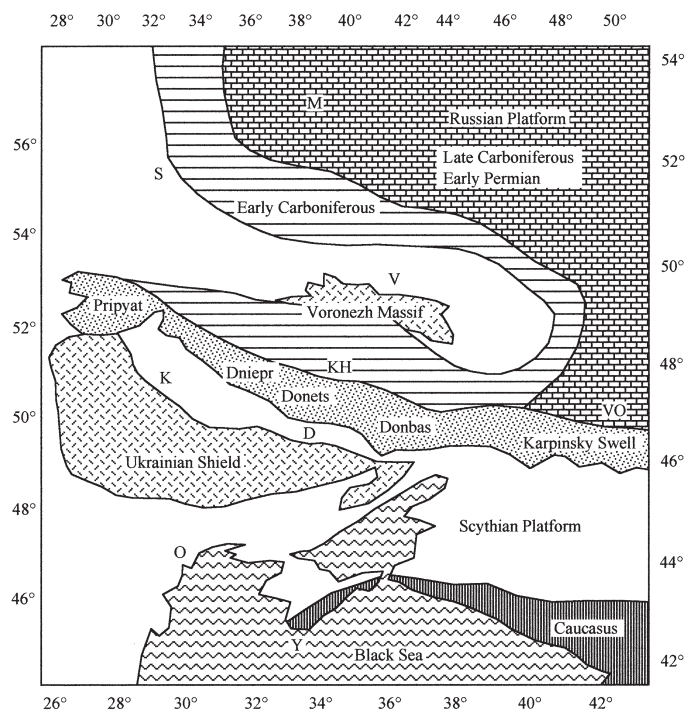
FIG. 1. – Location map showing the Moscow and Pripyat-Dniepr-Donets-Donbas basins. D : Donetsk, K : Kiev, KH : Kharkov, M : Moscow, O : Odessa, S : Smolensk, V : Voronezh, VO : Volgograd, Y : Yalta. FIG. 1. – Carte de localisation des bassins de Moscou et du Pripyat-Dniepr-Donets-Donbass
