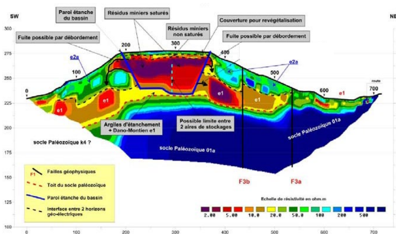
Figure 2. Coupe verticale du stockage de Montredon – Mise en évidence de matériaux pollués au sein de la digue Est
