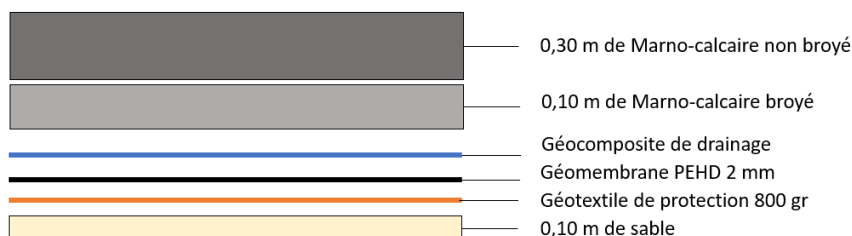
Figure 5. Coupe verticale et prise de vue de la nouvelle structure d'étanchéité
