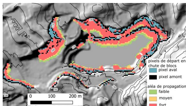
Figure 2 : Exemple des résultats fourni par ELANA à partir du MNT 5 m d'une ancienne carrière et d'un raster de même dimension où l'utilisateur déclare les pixels de départ en chute de blocs. ELANA classe les pixels de départ en pixels « amont » et « aval » et permet d'obtenir le raster des zones de propagation faible, moyenne et fortes à partir des lois empiriques proposées.
