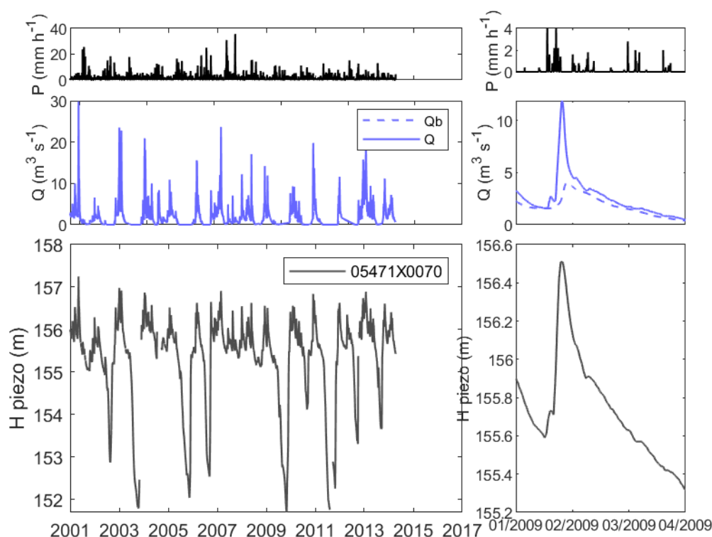
Figure 14 : Chronique des débits de l'Airain (Crosses - K554301001) et de la piézométrie au piézomètre 05471X0070 - Vornay . Source des données : Météo France, Banque Hydro et ADES / BRGM.
