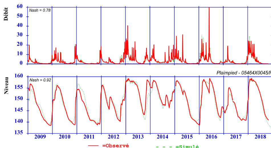
Figure 29 : Simulations du débit moyen journalier de l'Auron à Ormediot (K5653010) et de la piézométrie au piézomètre de Plaimpied (05464X0045/P) obtenues à l'aide de l'outil GARDÉNIA :
