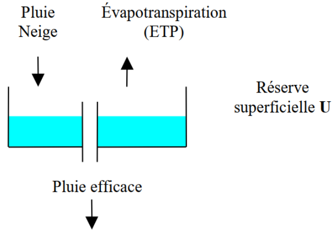
Figure 2 : Réservoir sol de type "réserve utile" (tout ou rien) (Thiery, 2014).
