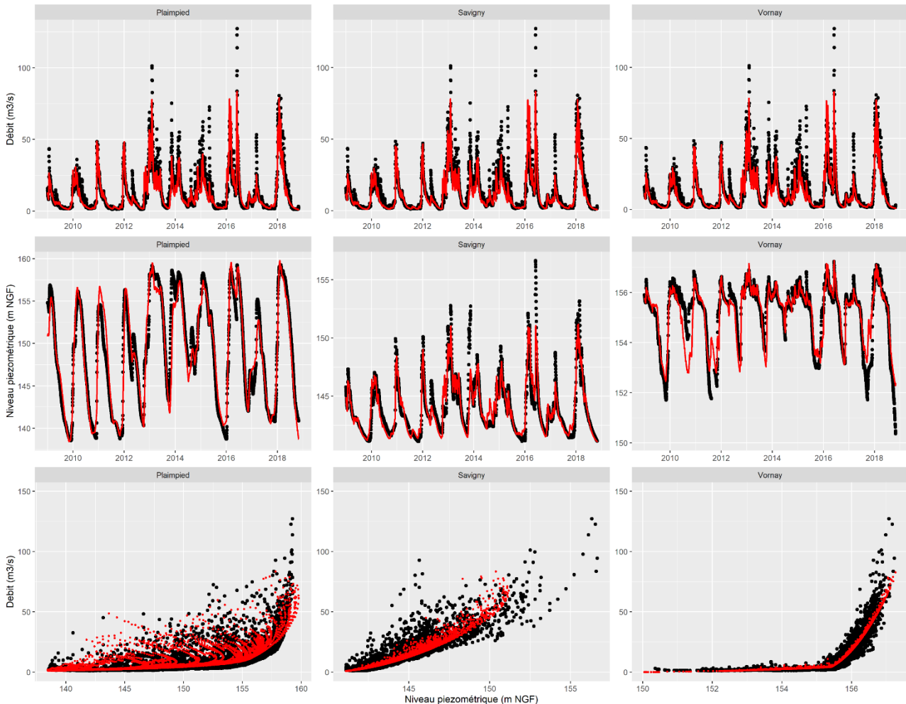
Figure 33 : Simulations pluie-débit-piézométrie du débit journalier de l'Yèvre à Saint Doulchard (Bourges) et dans trois piézomètres du bassin de l'Yèvre. Les simulations sont en rouge, les observations sont en noir.
