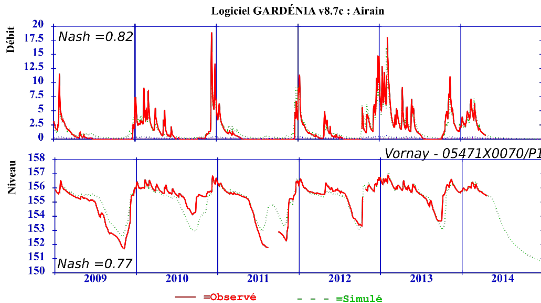
Figure 28 : Simulations GARDÉNIA du débit moyen journalier (haut) de l'Airain à Crosses (K5543010) et de la piézométrie (bas) au piézomètre de Vornay (05471X0070/P1) obtenues avec GARDÉNIA.
