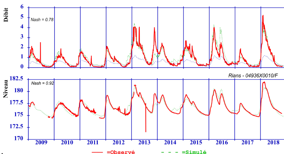
Figure 30 : Simulations du débit moyen journalier de l'Ouatier à Moulins sur Yèvre (Maubranche - K5554580) et de la piézométrie au piézomètre de Rians (04936X0010/F) obtenues avec GARDÉNIA.
