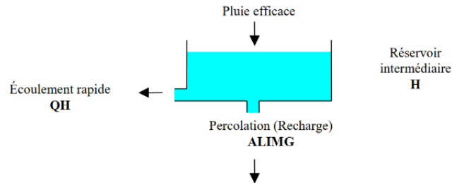
Figure 3 : Schéma du réservoir intermédiaire H (Thiery, 2014).
