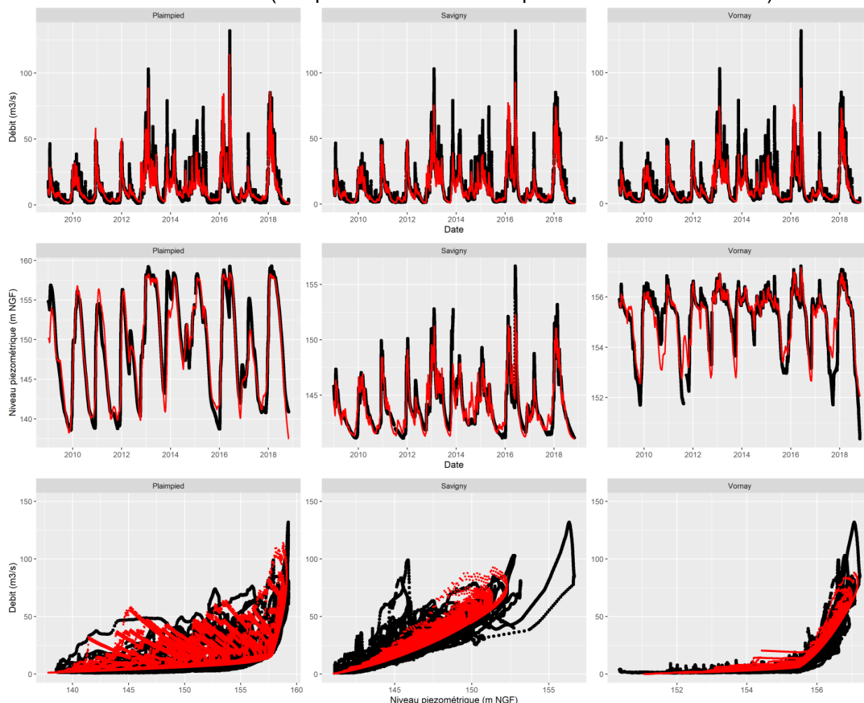
Figure 34 : Simulations pluie-débit-piézométrie du débit horaire de l'Yèvre à Saint Doulochard (Bourges) et dans trois piézomètres du bassin de l'Yèvre. Les simulations sont en rouge, les observations sont en noir. Haut : débits. Milieu : piézométrie. Bas : relations débit- piézométrie.
