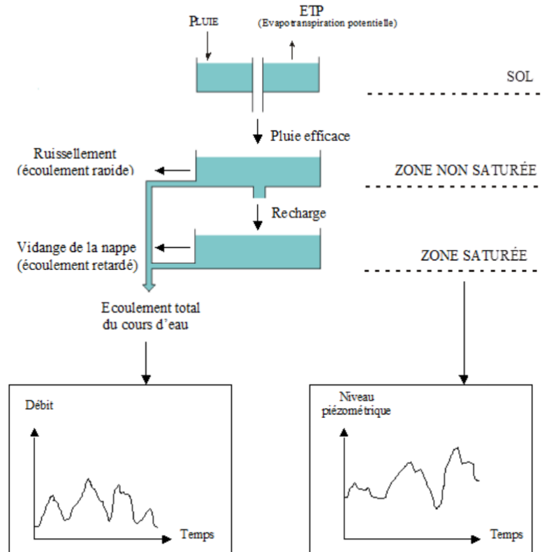
Figure 1 : Structure simple du modèle GARDENIA simple pour la simulation des débits de rivière et de niveaux de nappe (Thiery, 2014).
