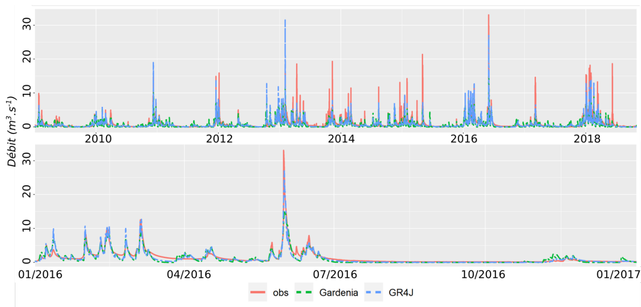
Figure 32: Comparaison des simulations GARDENIA et GR4J au pas de temps horaire sur le bassin du Moulon. Haut : Chronique complète. Bas : Détail du premier semestre 2016.
