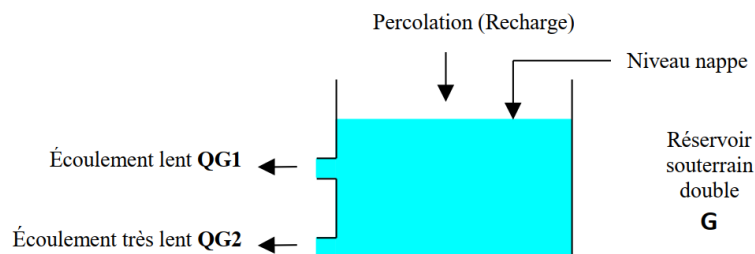
Figure 6 : Structure du réservoir souterrain à seuil G (Thiery, 2014).
