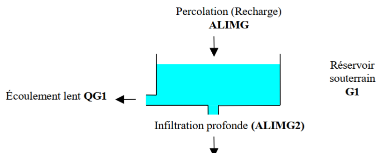
Figure 4 : Structure du réservoir souterrain G1 (Thiery, 2014).
