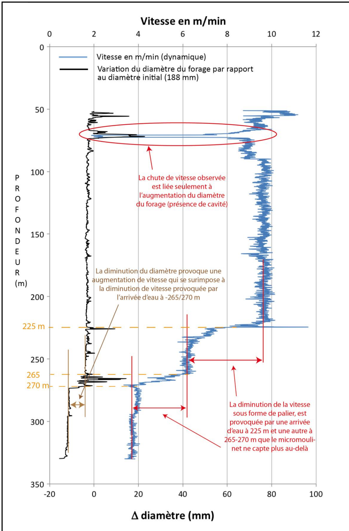
Illustration 6 : Diagraphie sur le forage du Triadou - vitesse mesurée par un micromoulinet lors d'un écoulement forcé (pompage à 15,8 m 3 /h) et variation du diamètre du forage par rapport à un diamètre initial de 188 mm
