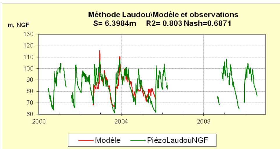
Figure 16 : Méthode de transfert du piézomètre «Laudou» : comparaison de la piézométrie simulée et observée. Les données observées depuis 2008 sont celles de la sonde automne Diver installée par Université de Gottingen dans le cadre du programme Pumpink
