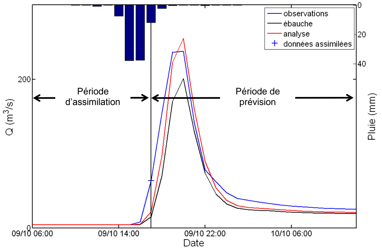
Figure 105 : Hydrogrammes observé (courbe bleue), simulé à partir de l'ébauche S^b = 160 mm (courbe noire) et simulé à partir de l'analyse S^a = 131 mm (courbe rouge) après assimilation d'une donnée (croix bleue) pour l'épisode d'octobre 2001. Le trait vertical noir sépare la période d'assimilation de la période de prévision
