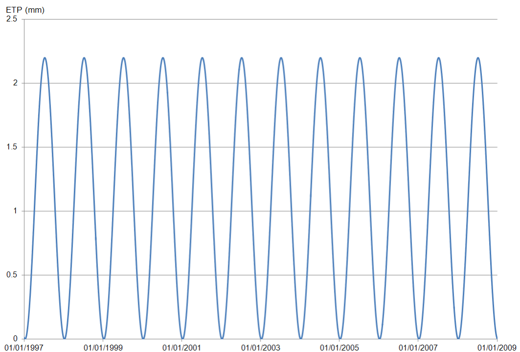
Figure 24 : ETP sinusoïdale
