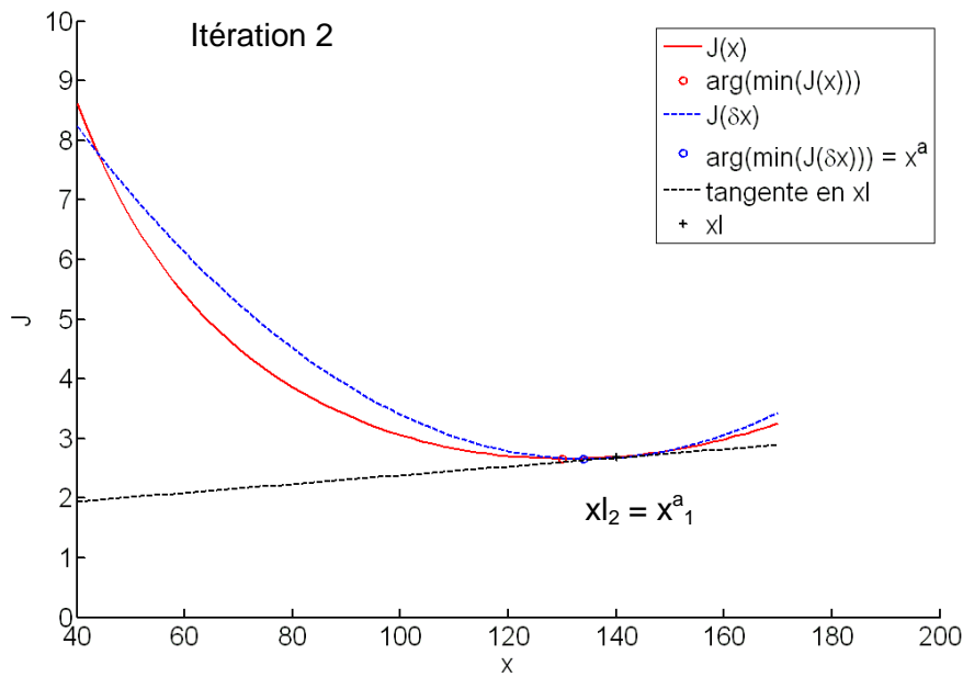
Figure 106 : Graphiques représentant la fonction coût J(\mathbf{x}) (courbe rouge) et son minimum (rond rouge) ainsi que l'évolution de la fonction coût incrémentale J(\mathbf{x}_l; \delta \mathbf{x}) (courbe bleue), de son minimum \mathbf{x}^a (rond bleu) et de sa tangente (droite noire) au point de linéarisation \mathbf{x}_l (croix noire) pour les 2 premières itérations de la boucle externe pour l'épisode d'octobre 2001
