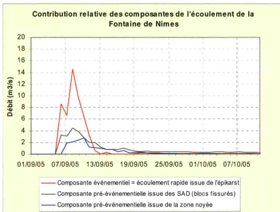
Illustration 30 : Décomposition des différentes composantes de l'hydrogramme de la Fontaine de Nîmes pour l'épisode de septembre 2005
