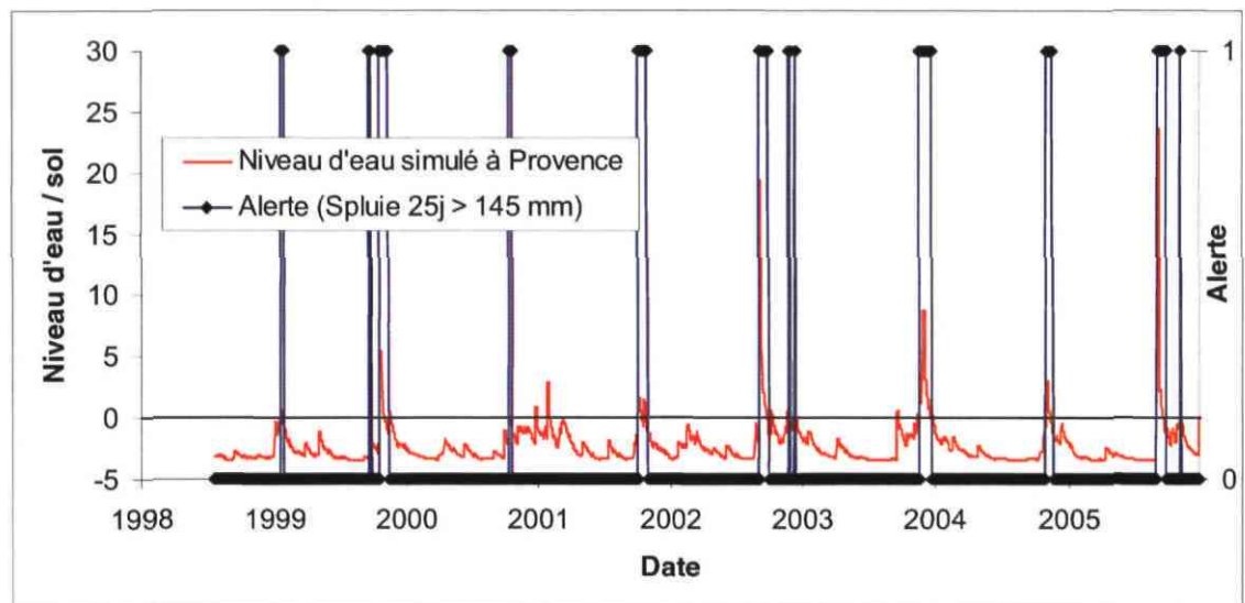
Illustration 51 : Niveau d'eau simulé à Provence par rapport au sol et déclenchement d'alerte pour un cumul de pluie sur les 25 jours précédents supérieur à 145 mm
