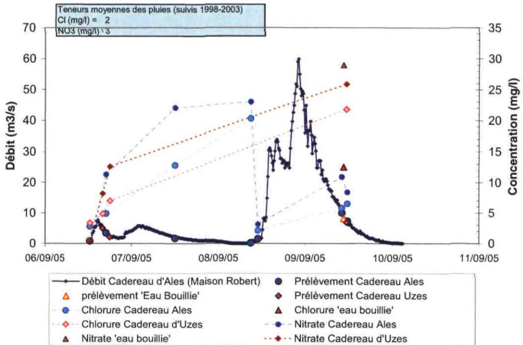
Illustration 72 : Evolution temporelle des débits mesurés à la fontaine de Nîmes et au cadereau d'Alès (Maison Robert) et des concentrations en chlorure (Cl) et en nitrate (NO3) mesurées dans les eaux.
