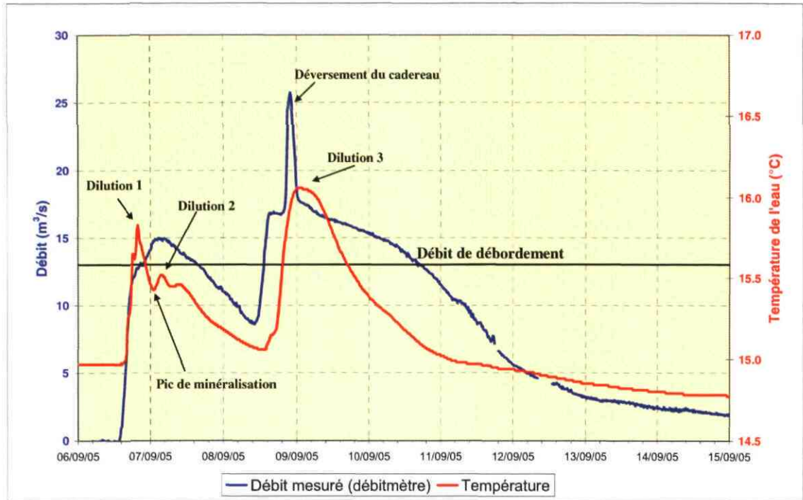
Illustration 24 : débit et température à la Fontaine de Nîmes durant la crue de septembre 2005
