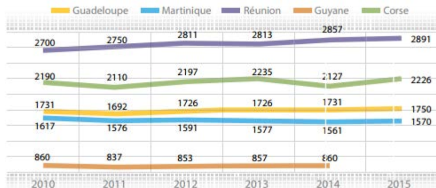
Figure 4 : Production d'électricité dans les ZNI en GWh
