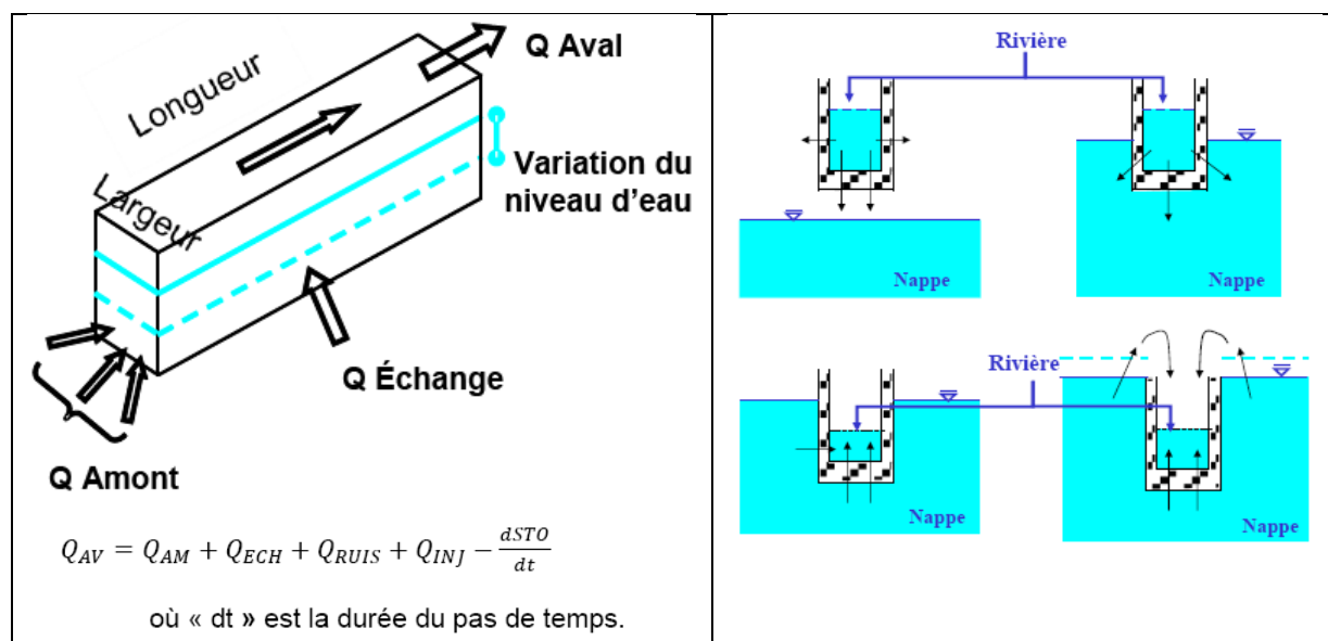
Figure 2 – Bilan des débits dans un tronçon de rivière et différentes configurations d'échange modélisées par MARTHE (Thiéry, 2015)
