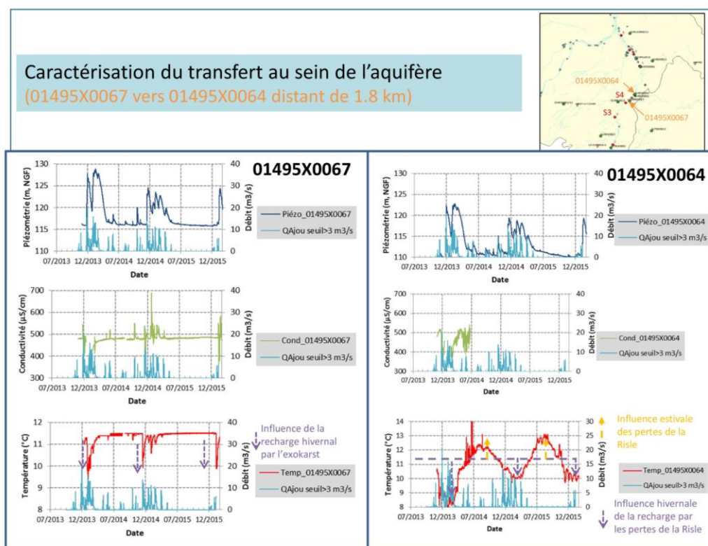
Figure 7 : Examen des évolutions des niveaux, de la minéralisation et de la température de l'eau souterraine au voisinage des ouvrages 01495X0067 (amont hydraulique de la Bétoire d'Ajou) et 01495X0064 (piézomètre à proximité de la Bétoire d'Ajou) (David et al., 2017)
