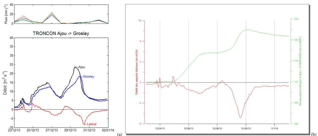
Figure 6 : (a) simulation des échanges latéraux sur le tronçon Ajou-Grosley lors du passage de la crue de décembre 2013 (les valeurs de débit négatif illustrent des pertes, et les valeurs positives des apports latéraux) ; (b) comparaison des échanges latéraux simulés sur le tronçon Ajou-Grosley (en rouge) et du niveau piézométrique mesuré dans le karst à Ajou sur le piézomètre 01495X0064 (David et al., 2017)
