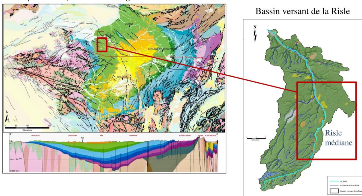
Figure 1 : Localisation de la Risle médiane au sein du bassin parisien (présentation BRGM – 22 ème journées technique du Comité Français d’Hydrogéologie de l’AIH : Hydrogéologie de la craie - Le Havre 2018)
