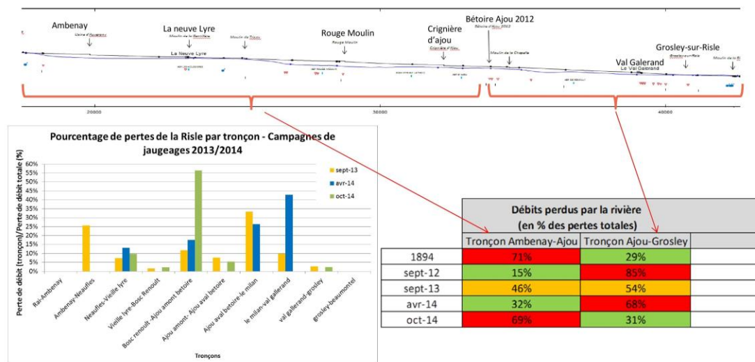
Figure 5 : Répartition et localisation des pertes de débits le long de la Risle médiane (David et al., 2017)
