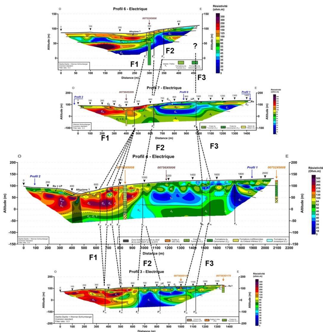
Figure 5 : Corrélation des profils géo-électriques orthogonaux à la faille de Fécamp-Lillebonne qui met clairement en évidence sa structure en faisceaux
