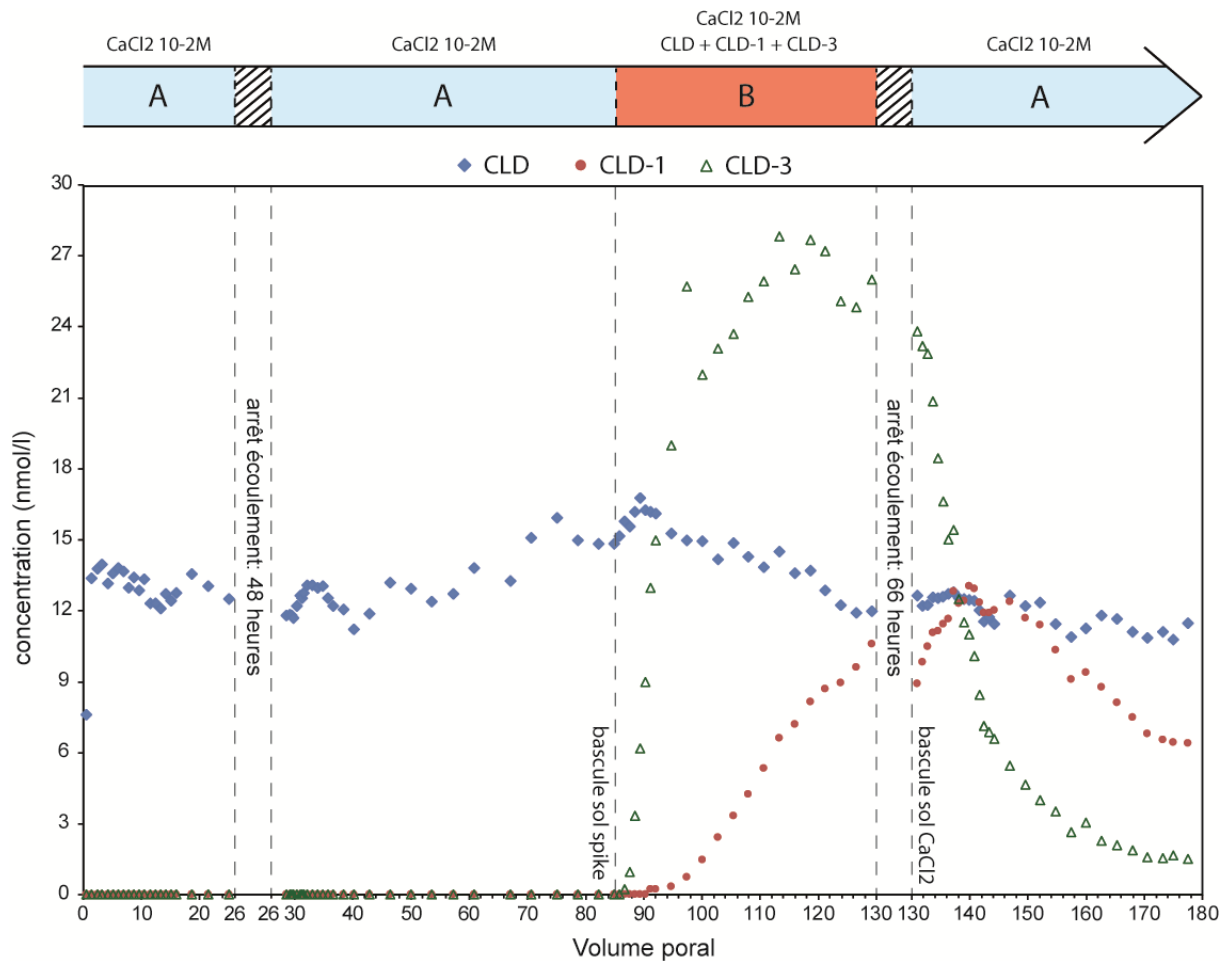
Evolution des concentrations en sortie de colonne de la CLD, CLD-1Cl et la CLD-3Cl en fonction de la nature de la solution injectée (A: CaCl 2 10 -2 M; B: CaCl 2 10 -2 M + CLD, CLD-1Cl + CLD-3Cl, cf texte pour détails) et des arrêts éventuels de l'injection.
