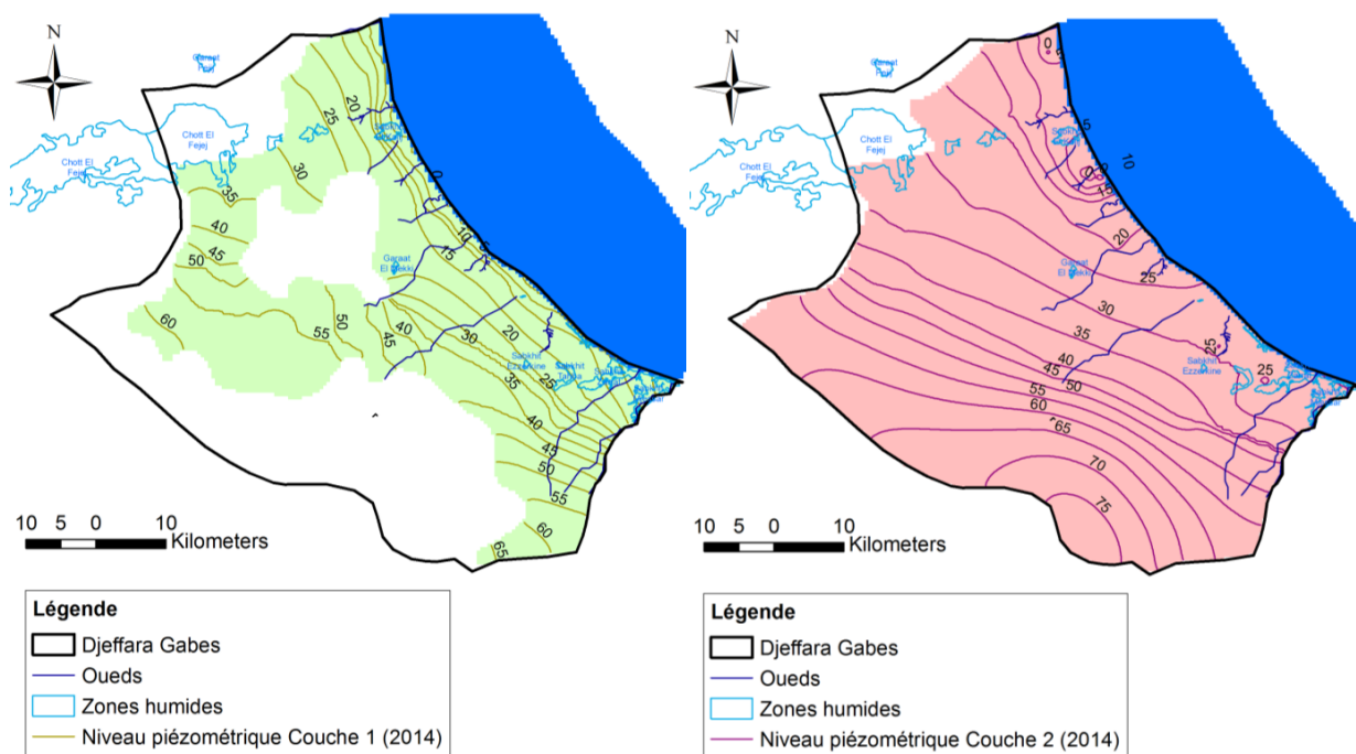
Figure 4. Cartes piézométriques simulées en 2014
