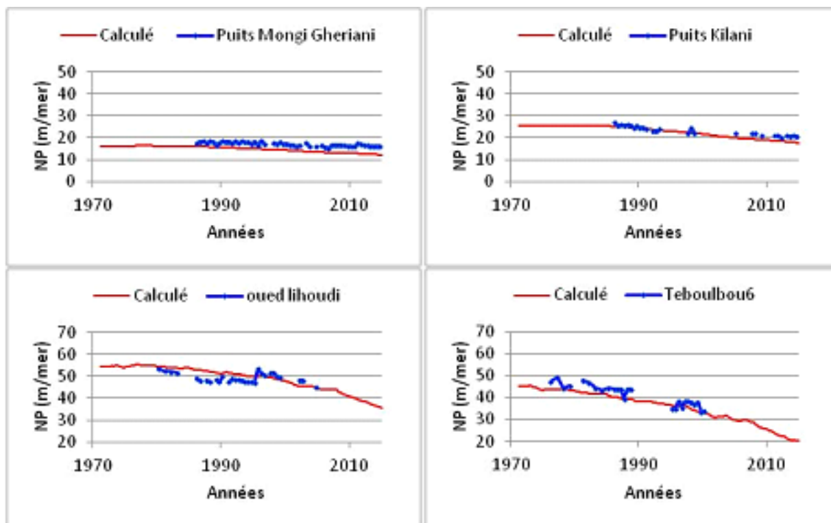
Figure 2. Evolution des niveaux piézométriques mesurés et calculés
