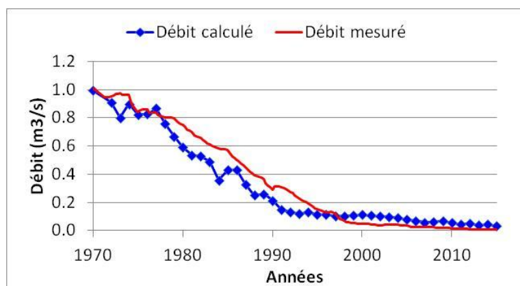
Figure 3. Evolution du débit des sources
