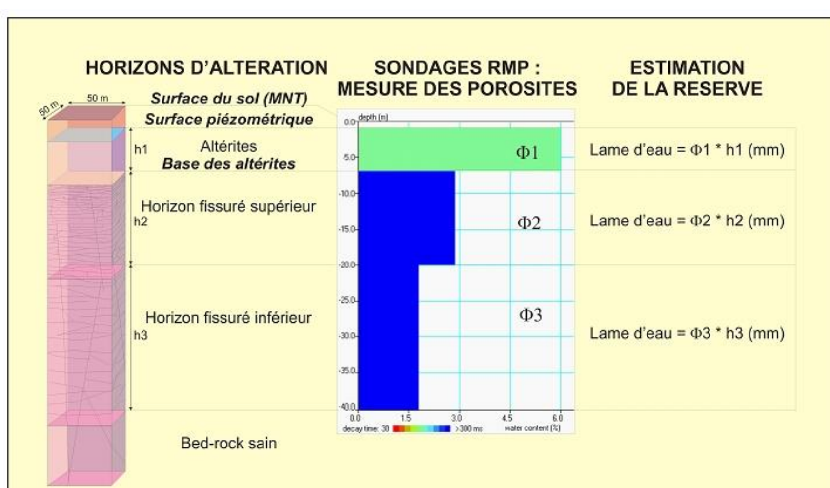
Organigramme de réalisation de la carte de la réserve en eau souterraine (Wyns et al. 2004)
