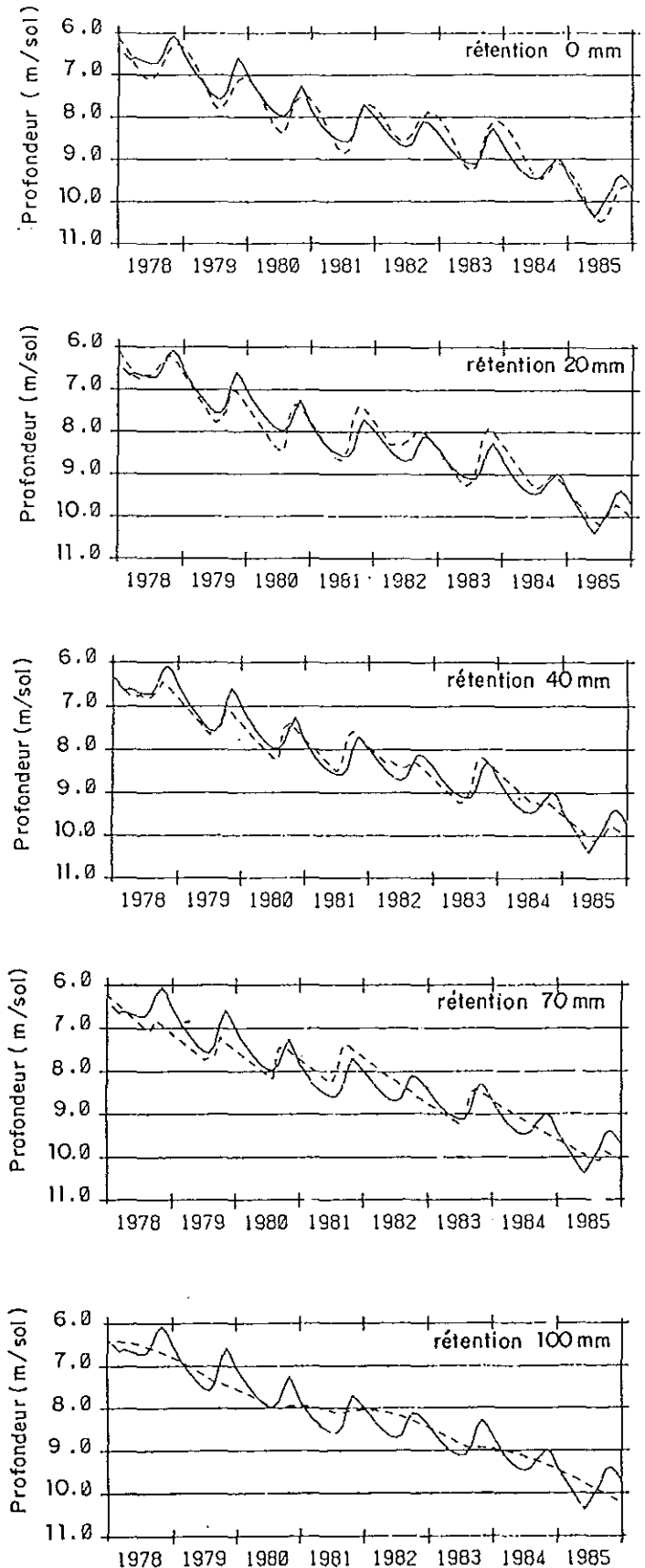
Fig. 4 - Simulation des niveaux avec une capacité de rétention de 0 à 100 mm — niveaux observés ---- niveaux calculés
