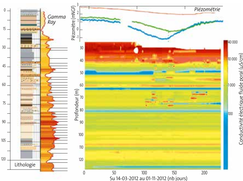
▲ Profil de conductivité électrique du fluide poral au regard de la piézométrie ainsi que du log lithologique et du gamma ray à Barcarès (plaine du Roussillon). En rouge, dans la zone comprise entre 60 et 80 mètres de profondeur, augmentation de la salinité après 100 jours et en orange, dans la zone supérieure à 110 mètres après 150 jours.
