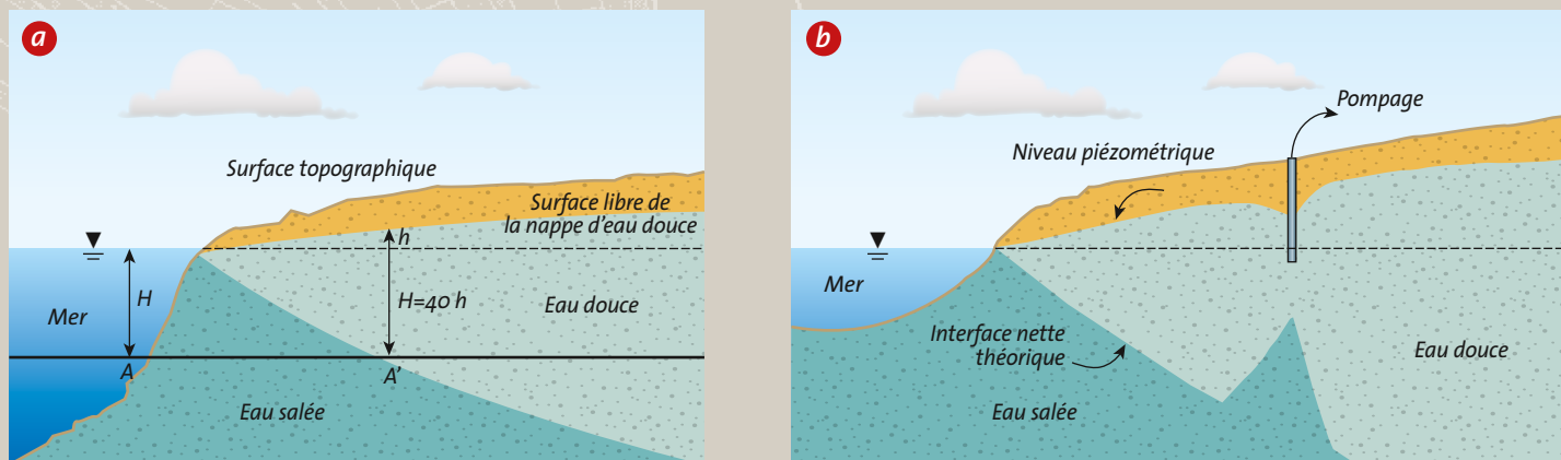
▲ Fig. 1 : (a) Coupe schématique perpendiculaire au littoral selon le principe de Ghyben-Herzberg et (b) Impact d'un pompage sur l'interface eau douce/eau salée selon le principe de Ghyben-Herzberg.
