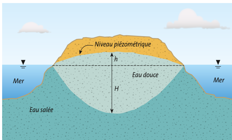
▲ Fig.3 : Schéma d'un aquifère insulaire.
