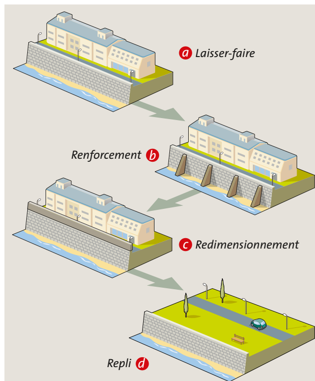
▲ Fig. 1 : Stratégies d'adaptation à l'élévation du niveau marin. Fig. 1: Strategies of adaptation to mean sea level rise. © CETMEF.
