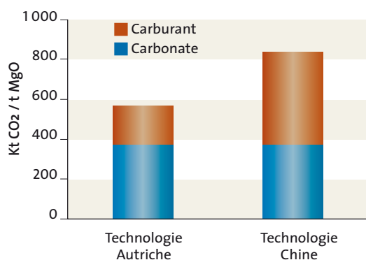
▲ Fig. 4 : Émissions de CO 2 par tonne de magnésium produite (Drnek, 2008).
