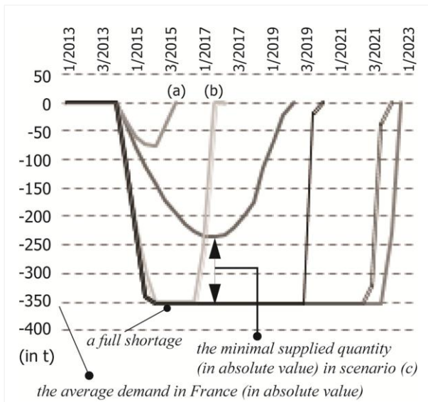
FIG. 3 - Evolution prospective du stock de lithium en France
