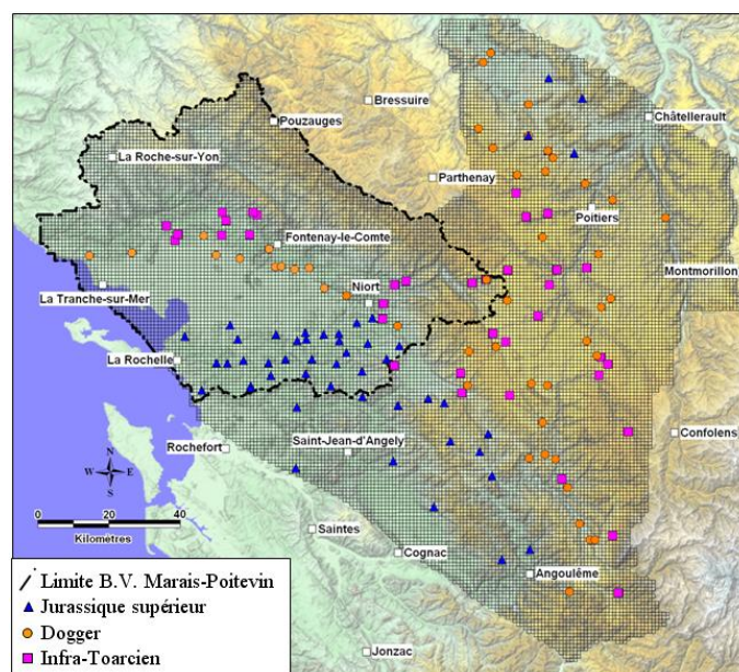
Figure 3 – localisation des piézomètres utilisés
