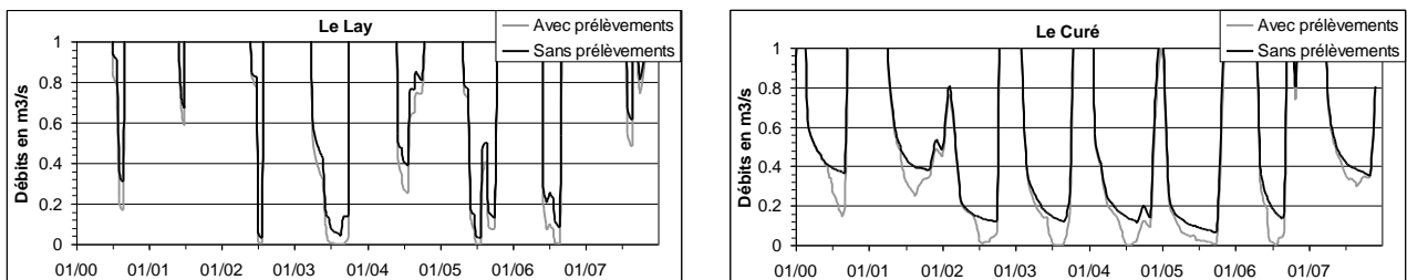
Figure 12 – débits simulés des cours d'eau à l'entrée du Marais Poitevin (sur des points fictifs) avec prélèvements (calage) et sans prélèvement
