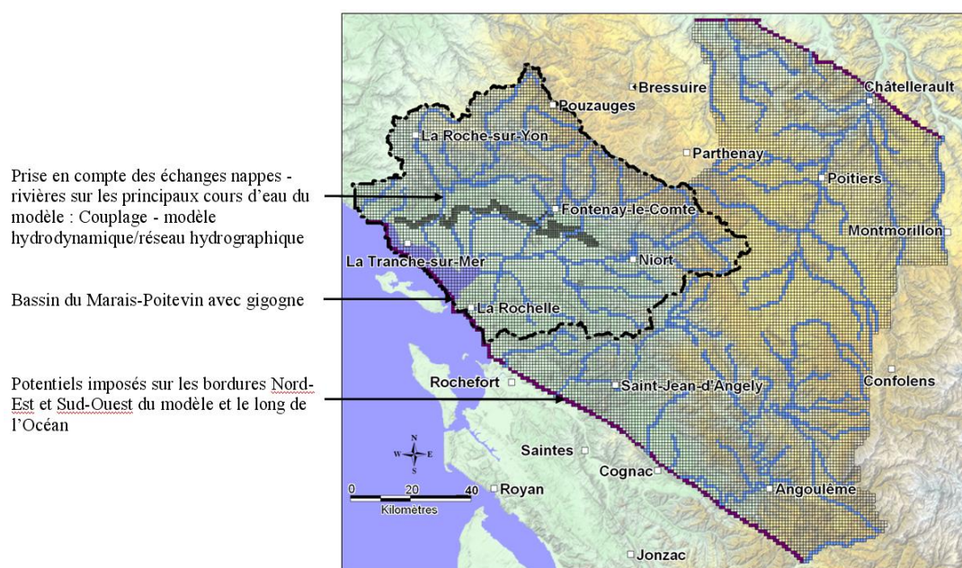
Figure 2 – extension du modèle : cours d'eau et potentiels imposés intégrés dans le modèle
