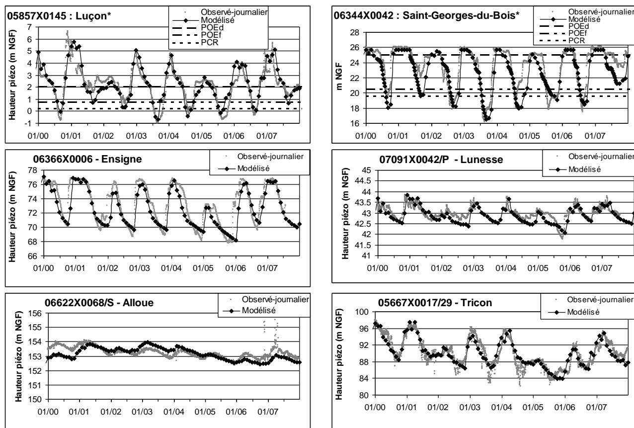
Figure 4 – comparaison des chroniques piézométriques observées/simulées (* exemple sur le secteur du Marais)
