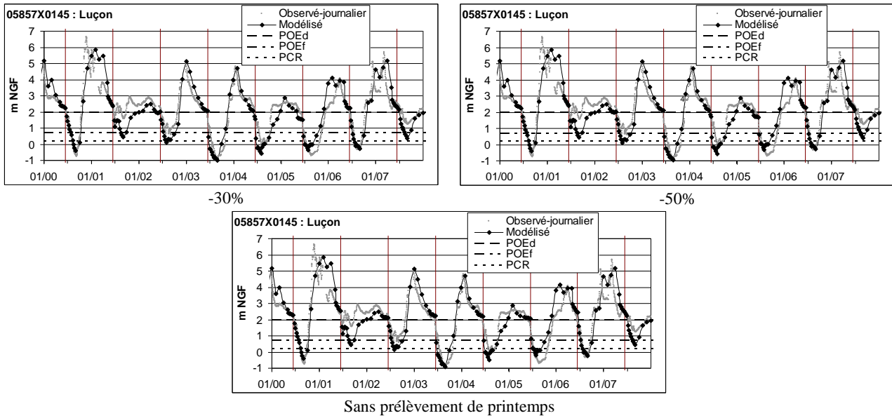
Figure 10 – graphiques de résultats des simulations de baisse de prélèvements sur la période de printemps (avril-15 juin)
