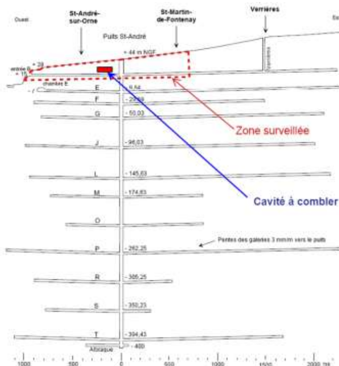
Figure 2 : Vue en coupe (ouest-est) du flanc nord et des travaux miniers
