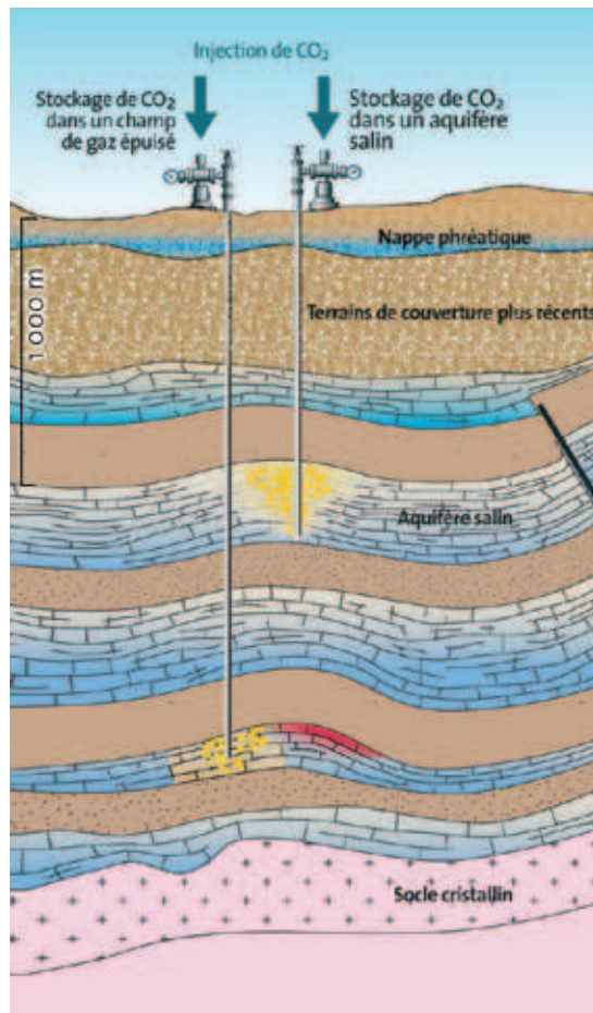
Fig. 3 : Schéma du stockage de CO 2 en couches géologiques profondes.
