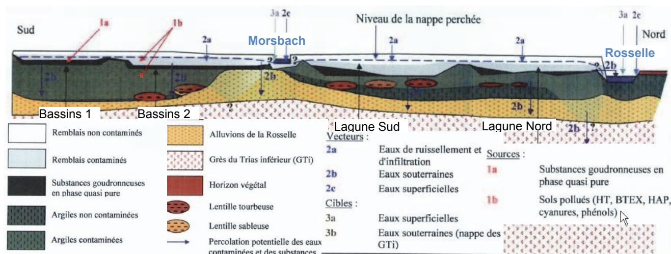
Figure 2. Coupe Sud Nord du site avant travaux
