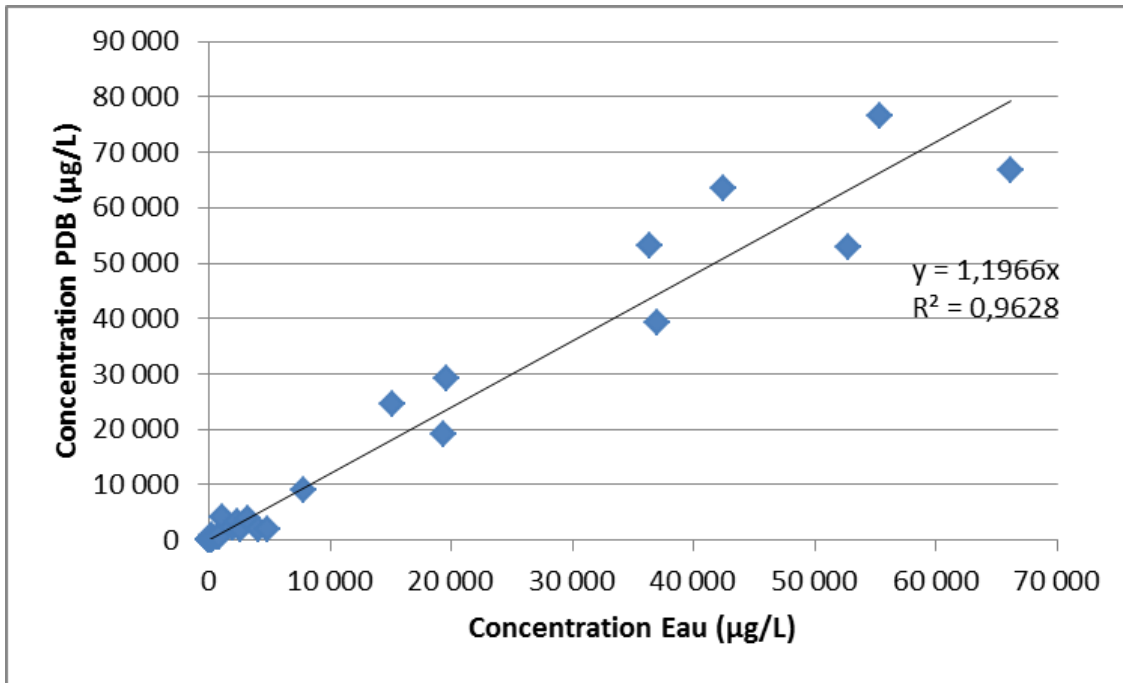
Figure 1 : Comparaison des concentrations obtenues à l'aide de PDB et de prélèvements multi-niveaux
