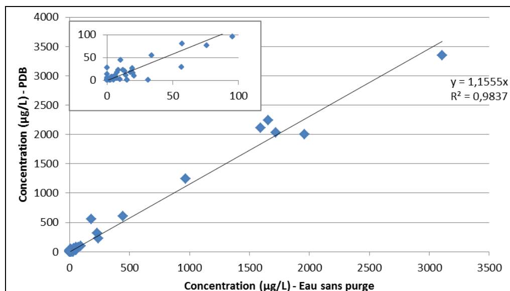
Figure 3 : Comparaison des concentrations obtenues avec PDB et prélèvement d'eau avant purge au retrait des échantillonneurs (de l'ordre de 60 mesures)
