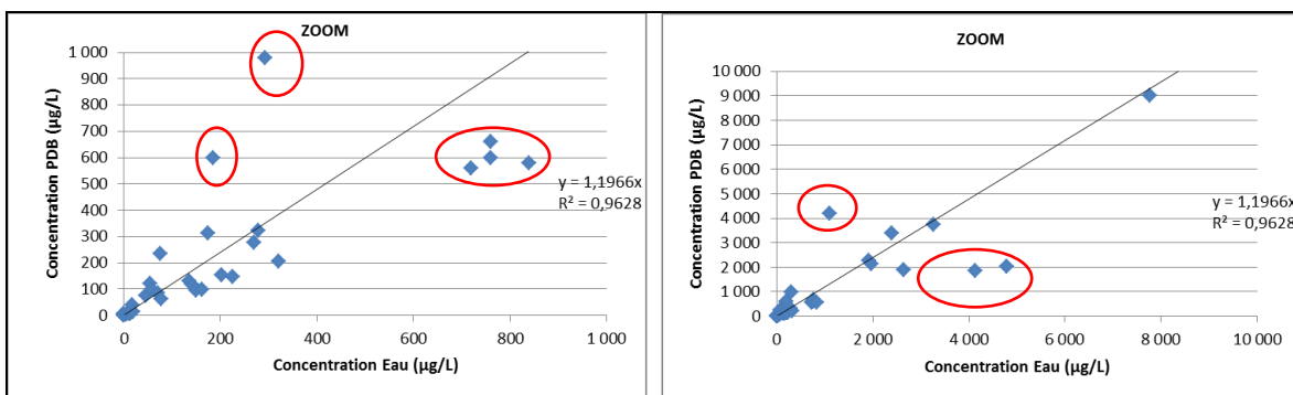
Figure 2 : Comparaison des concentrations obtenues à l'aide de PDB et de prélèvements multi-niveaux (zoom)
