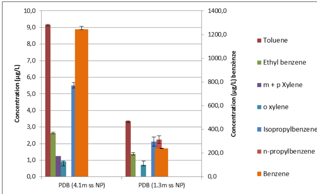
Figure 4 : Concentrations obtenues avec les PDBs à deux profondeurs (NP : Niveau piézométrique)
