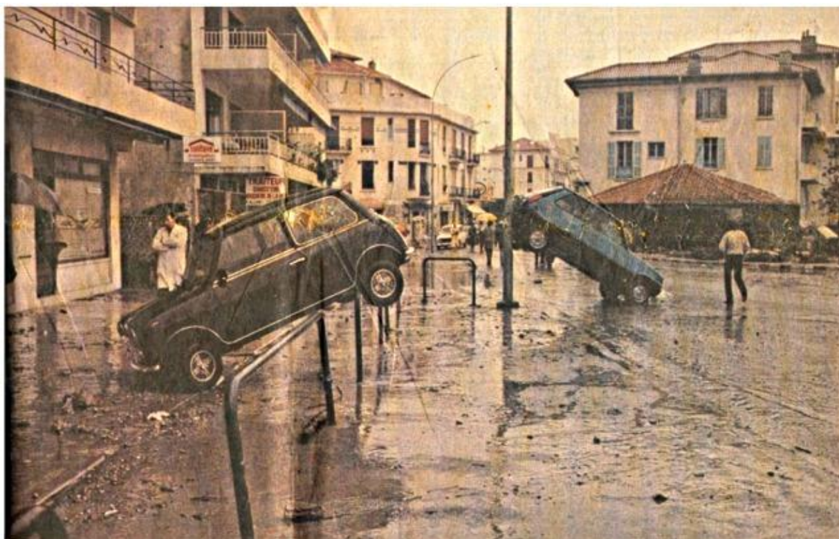
Figure 10: Photographie des conséquences du tsunami du 1979 à Antibes ( http://www.lamouettelaurentine.net/st_laurent_du_var/port/tsunami.htm ).
