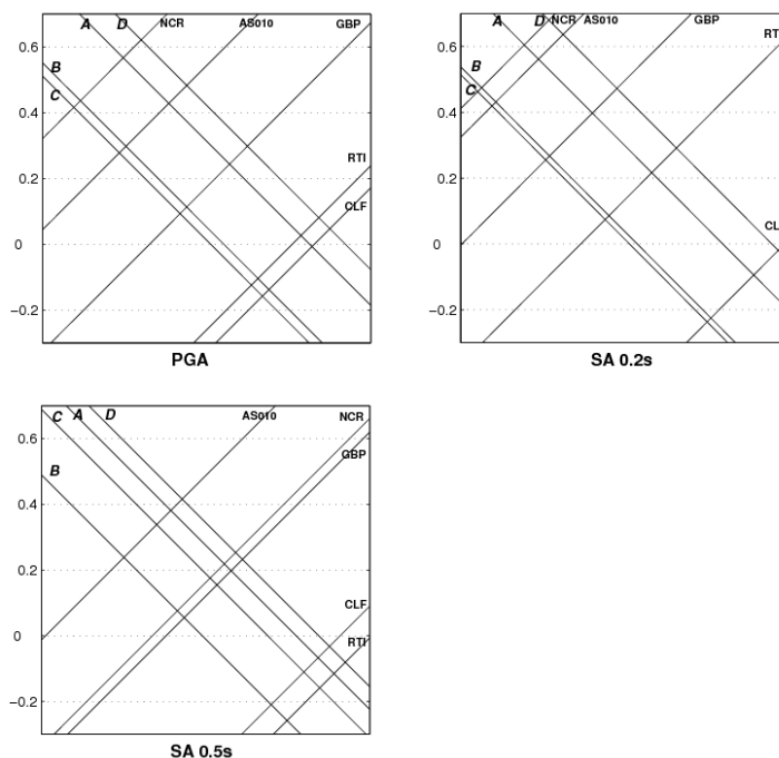
Figure 1. Régression linéaire à deux composantes pour les données issues de la séquence d'Ombrie de 1997-1998. Les nombres sur l'axe des ordonnées indiquent approximativement les résidus par rapport aux relations de prédiction de Ambraseys et al. (2005).
