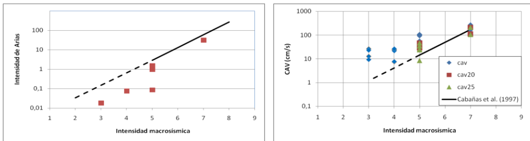
Figura 8 a) Valores de la Intensidad de Arias (AI) versus intensidad calculados para componentes horizontales de los acelerogramas registrados en el sismo de Lorca junto con la relación media establecida por Cabañas et al, 1997; b) Valores del parámetro CAV versus intensidad calculados para componentes horizontales de los acelerogramas registrados en el sismo de Lorca, junto con la relación media establecida por Cabañas et al., 1997
