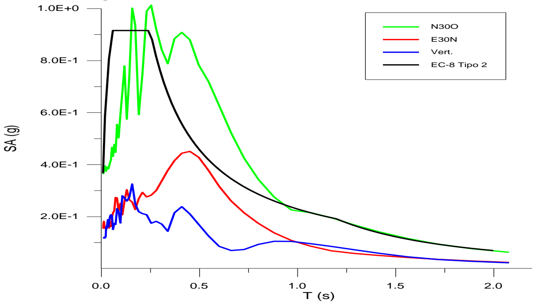
Fig. 12. Espectros de respuesta de las tres componentes de los acelerogramas registrados en Lorca junto con la forma espectral EC8 de tipo 2 para clase de suelo A (roca), escalado al PGA de 0,37g
