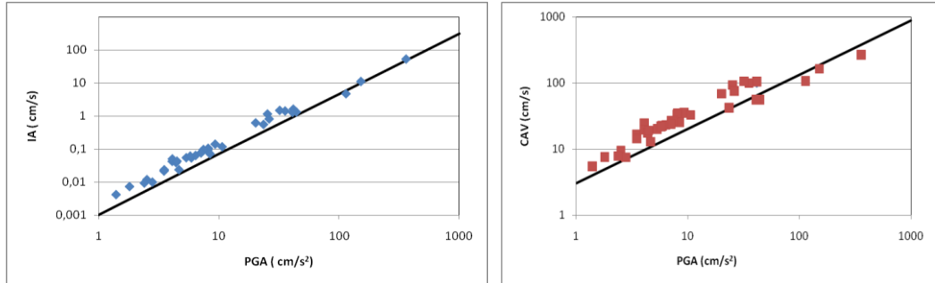
Fig. 3a AI vs PGA de todas las estaciones (componentes horizontales), junto a la recta de regresión obtenida de la base de datos europea NERIES (Oliveira et al., 2012); 3b CAV vs PGA de todas las estaciones (componentes horizontales), junto a la recta de regresión obtenida de la base de datos europea NERIES (Oliveira et al., 2012)
