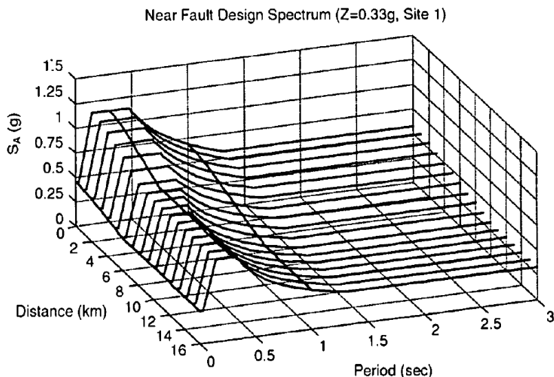
Fig. 13. Espectros de diseño para emplazamientos cercanos a la falla (Chai et al. 2000).
