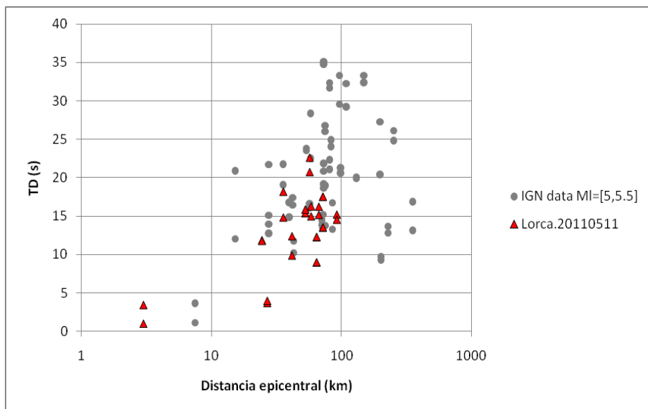
Fig. 5. TD versus distancia para el conjunto de acelerogramas registrados por la red del IGN para sismos de M5-5.5 (círculos). Los triángulos representan los valores obtenidos para el sismo de Lorca de M5.1
