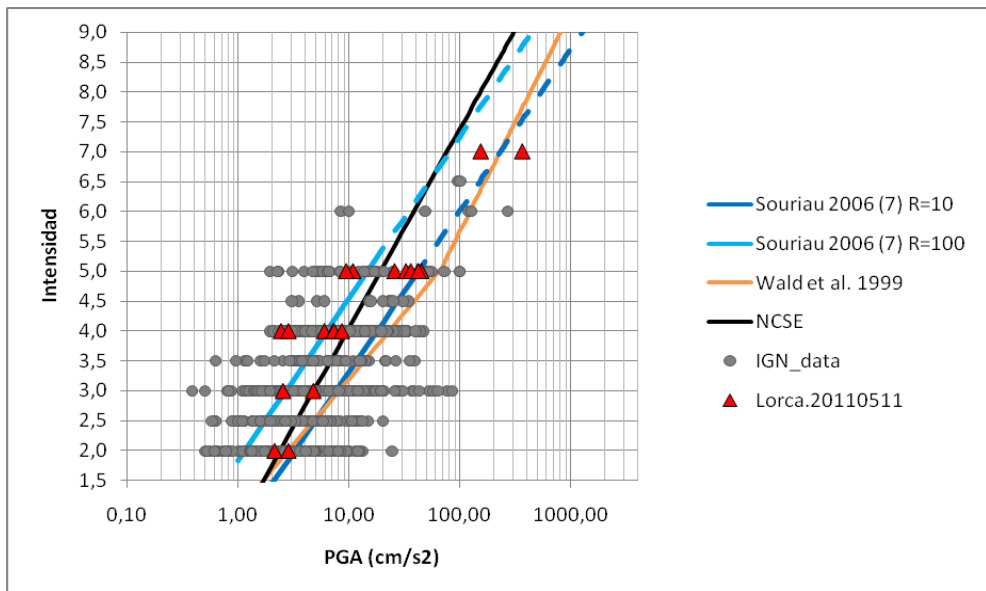
Fig. 7. Intensidades versus valores de PGA (componentes horizontales) observados para el conjunto de sismos existentes en la base de datos del IGN. En rojo, los puntos correspondientes a las observaciones del sismo de Lorca junto con las curvas de NCSE, Souriau (2006) y Wald et al. (1999).
