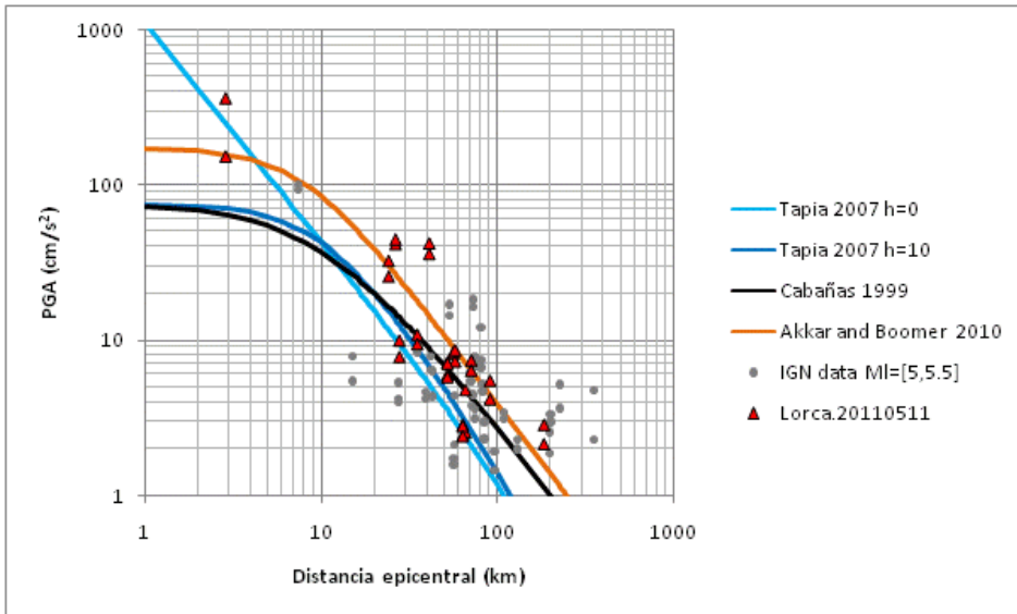
Fig. 4. PGA versus distancia para el conjunto de acelerogramas registrados por la red del IGN para sismos de M5-5.5 (círculos). Los triángulos representan los valores obtenidos para el sismo de Lorca de M5.1. Se representan curvas predictivas del movimiento del suelo (GMPE), según Tapia et al. (2007), Cabañas et al. (1999) y Akkar and Bommer (2010).
