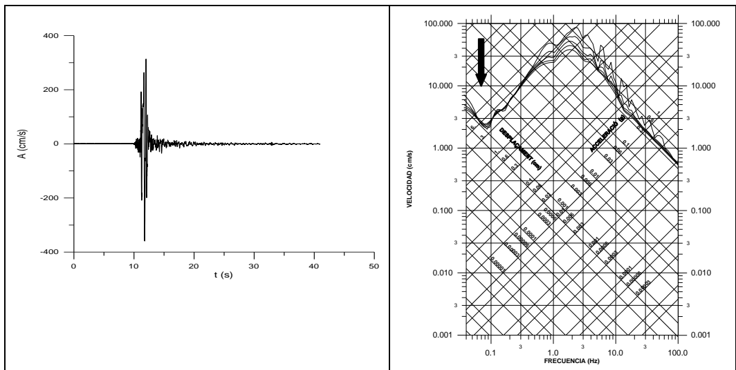
Fig. 2. Acelerograma corregido de línea de base y espectros de respuesta para distintos amortiguamientos asociados, correspondientes a la componente N30°O de la estación de Lorca del sismo principal. Se indica con una flecha la frecuencia de corte para el filtrado pasa –altas a 0,06Hz.
