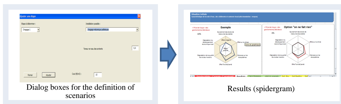
Figure 1. GeDseT tool
