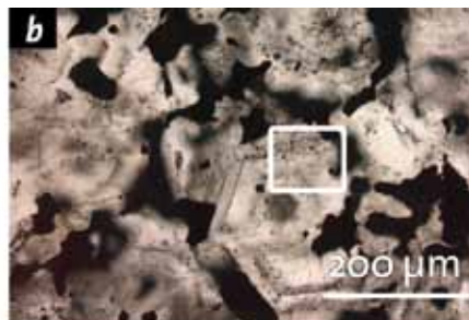
Inclusions fluides de la mine de cobalt, nickel, argent et or de Bou Azzer (2,5 Mt @ 1,27 % Co, 1 % Ni, 50 g/t Ag, 6 g/t Au) dans le sud du Maroc.
