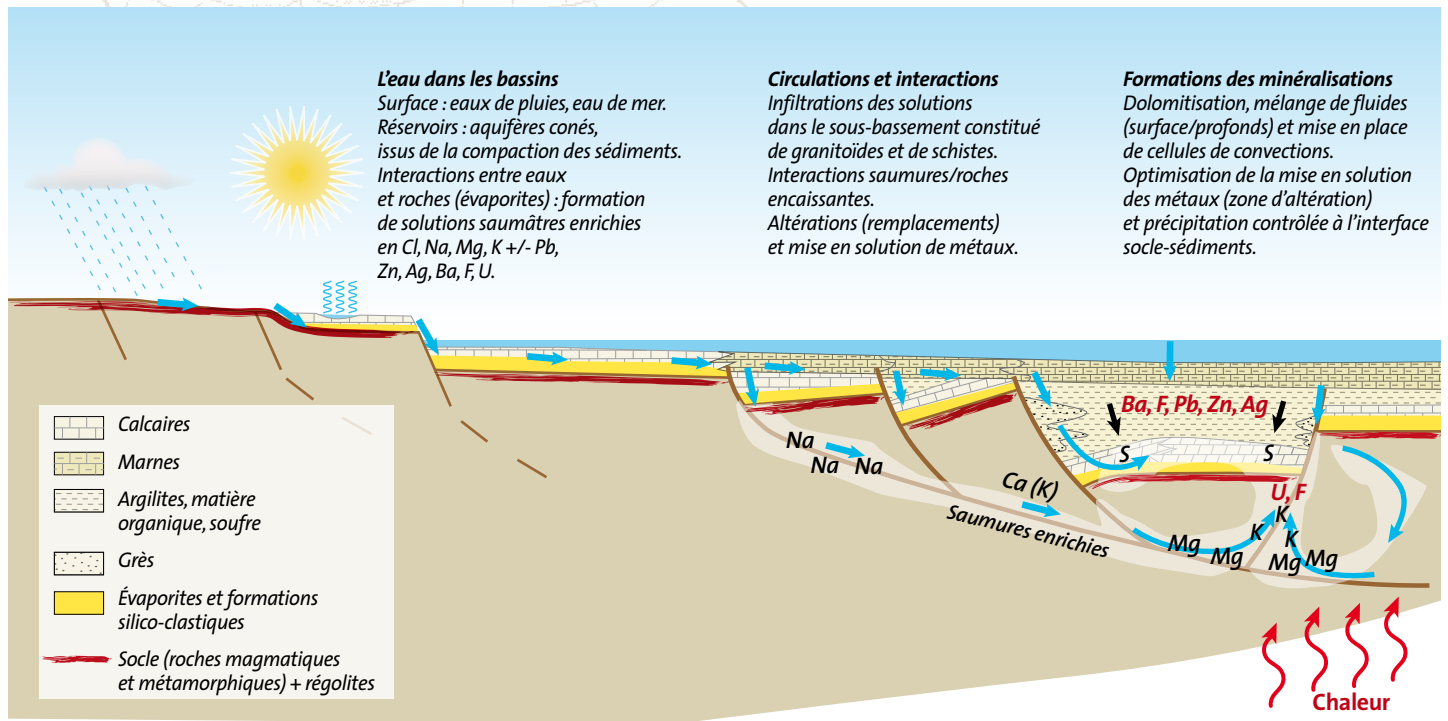
Fig. 3 : Les circulations de fluides à l'interface entre socle et couverture. Fig. 3: Fluid circulations at the interface between basement and cover.
