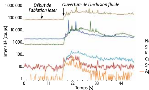
▲ Photographie de l'équipement d'ablation laser couplée à l'ICPMS (LA-ICPMS) installé au laboratoire G2R, Nancy. Photographie de l'inclusion fluide avant et après ablation. Spectre de masse obtenu après ablation laser et analyse d'une inclusion fluide.
