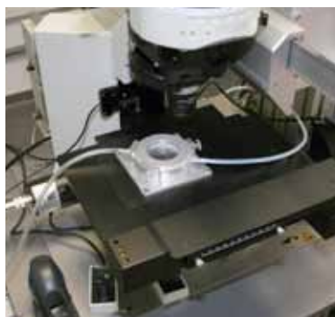
▲ Photographie de l'équipement d'ablation laser couplée à l'ICPMS (LA-ICPMS) installé au laboratoire G2R, Nancy. Photographie de l'inclusion fluide avant et après ablation. Spectre de masse obtenu après ablation laser et analyse d'une inclusion fluide.
