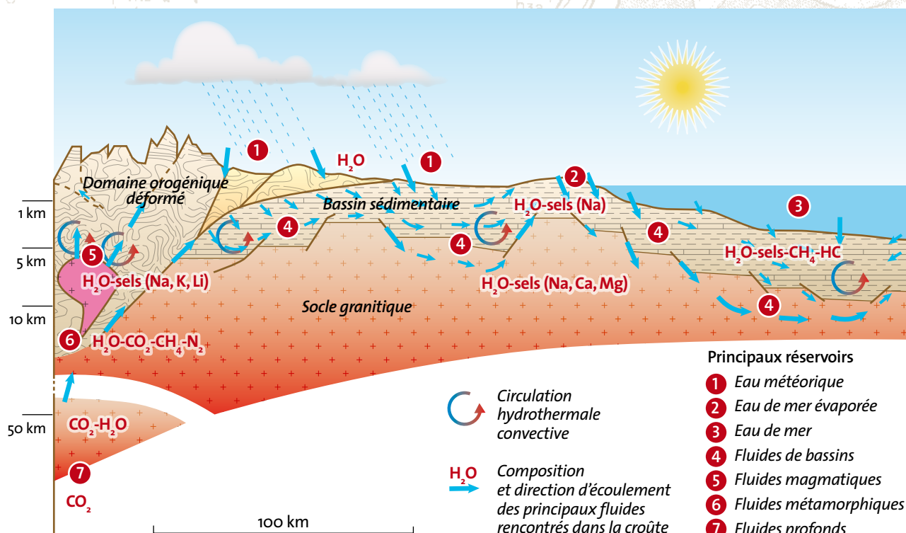
▲ Fig. 1 : Coupe présentant les principaux réservoirs fluides, les circulations des solutions hydrothermales et leurs compositions dans la croûte terrestre.
