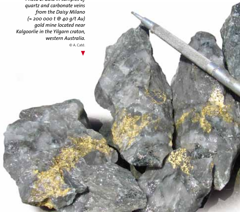
▶ Photo 2 : Or dans des échantillons de veines de quartz et carbonate de la mine d'or de Daisy Milano ( \approx 200\,000\text{ t} @ 40\text{ g/t Au} ) située près de Kalgoorlie dans le craton du Yilgarn en Australie occidentale.
