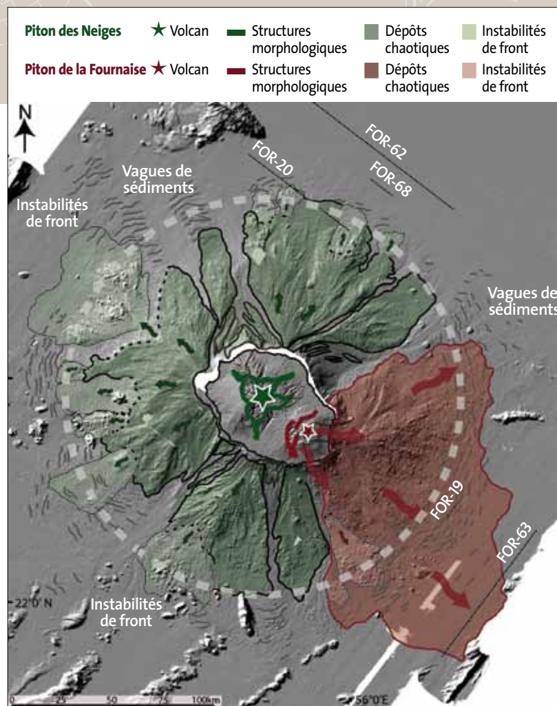
Fig. 4 : Modèle des glissements de flancs de l'île de la Réunion drapés sur les données bathymétriques et topographiques.
