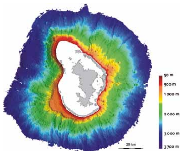
▲ Fig. 5 : À gauche : morphologie sous-marine de la pente insulaire (–200 à –3 500 m) de Mayotte montrant les transferts sédimentaires (canyons, glissements) et volcans isolés (Audru et al. , 2006). À droite : anomalies magnétiques (champ total réduit au pôle) montrant une structuration profonde WNW-ESE et anomalies magnétiques à très haute résolution de l'île.
