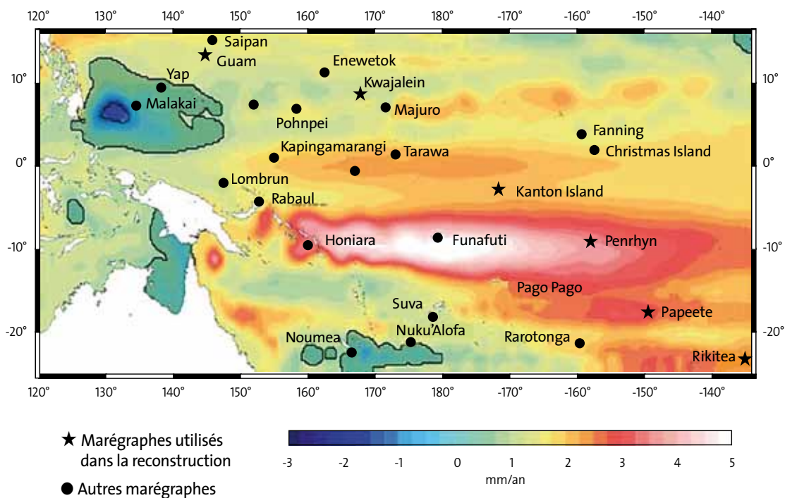
Fig. 1 : Tendances linéaires des variations du niveau marin dans le Pacifique tropical ouest, sur la période 1950-2009, reconstruites en utilisant des données marégraphiques et les modes de variabilité issus du modèle de circulation générale océanique DRAKKAR. D'après Becker et al. (2011).
