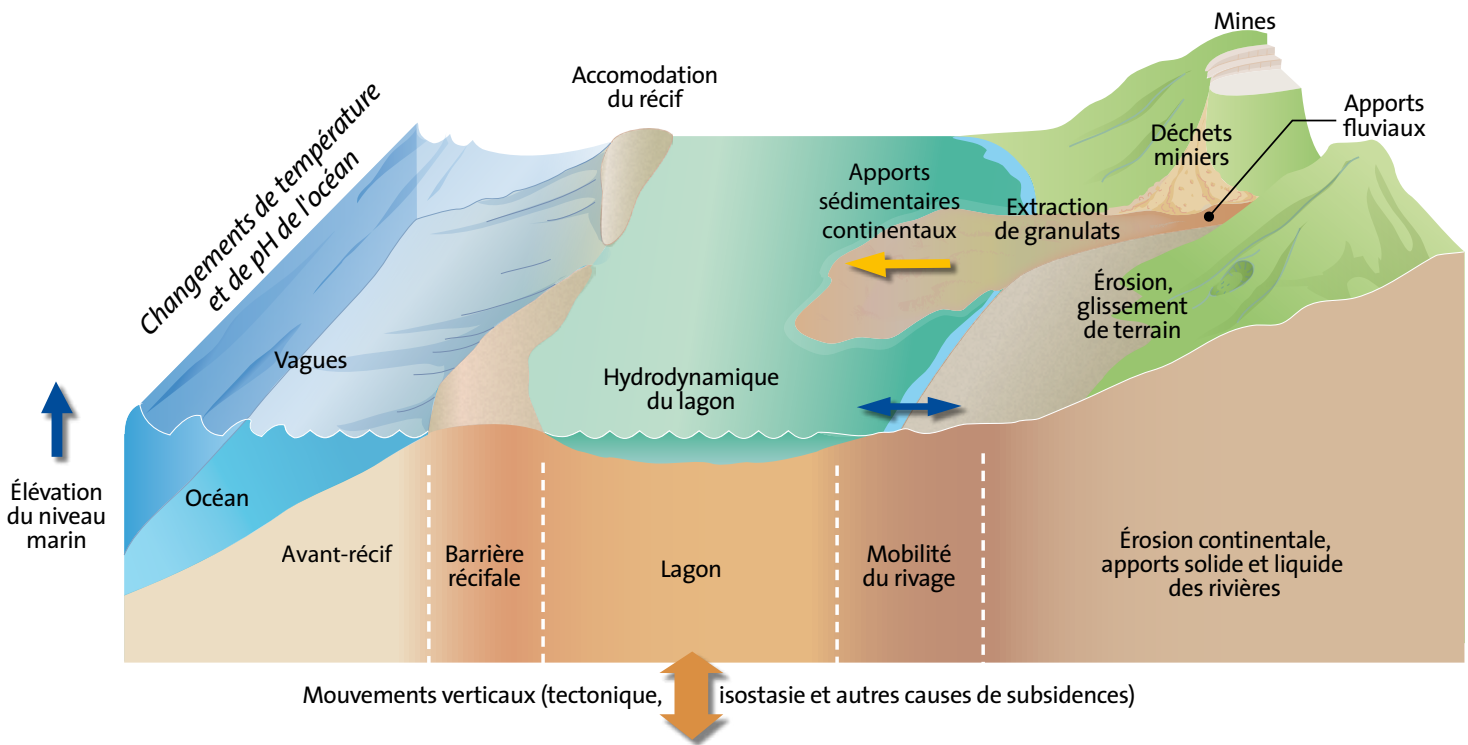
▲ Fig. 5 : Processus côtiers affectant la ligne de rivage d'un estuaire de Nouvelle-Calédonie.
