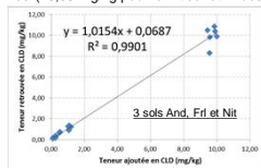
Figure 8 : Teneur retrouvée dans les sols après dopage à 0,1, 0,25, 0,5, 1 et 10 mg/kg sur Nitosol et Ferralsol et dopage à 1 et 10 mg/kg sur Andosol en doublet.
