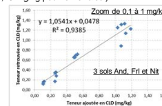
Figure 8 : Teneur retrouvée dans les sols après dopage à 0,1, 0,25, 0,5, 1 et 10 mg/kg sur Nitosol et Ferralsol et dopage à 1 et 10 mg/kg sur Andosol en doublet.
