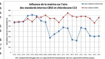
Figure 2 : Influence de la matrice sur l'aire des standards internes CB53 et chlordécone C13. La chlordécone 13 C est utilisée en standard interne puisque le PCB53 ne prend pas en compte les effets de matrice.
