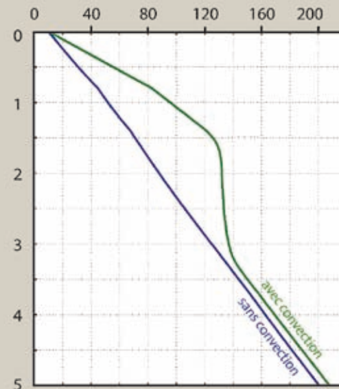
▲ Fig. 2 : En haut, données de température dans le graben du Rhin et profil mesuré à Soutz-sous-Forêts (trait plein) ; structure géologique simplifiée à droite. En bas, modèle numérique de convection hydrothermale. Le profil thermique obtenu en présence de convection (en vert) reproduit les mesures.
