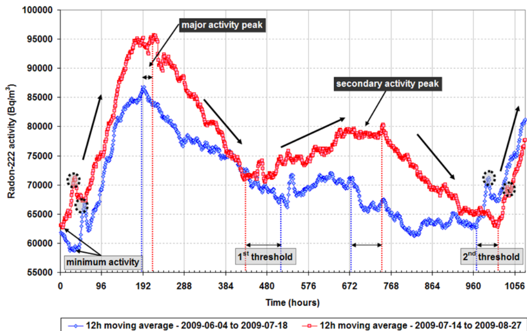
Figure 6 : Comparaison de deux cycles de 40 jours sur les activités radon. Comparison between two 40-days long radon activity cycles.
