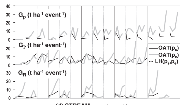
(d) STREAM - same key as (c)
